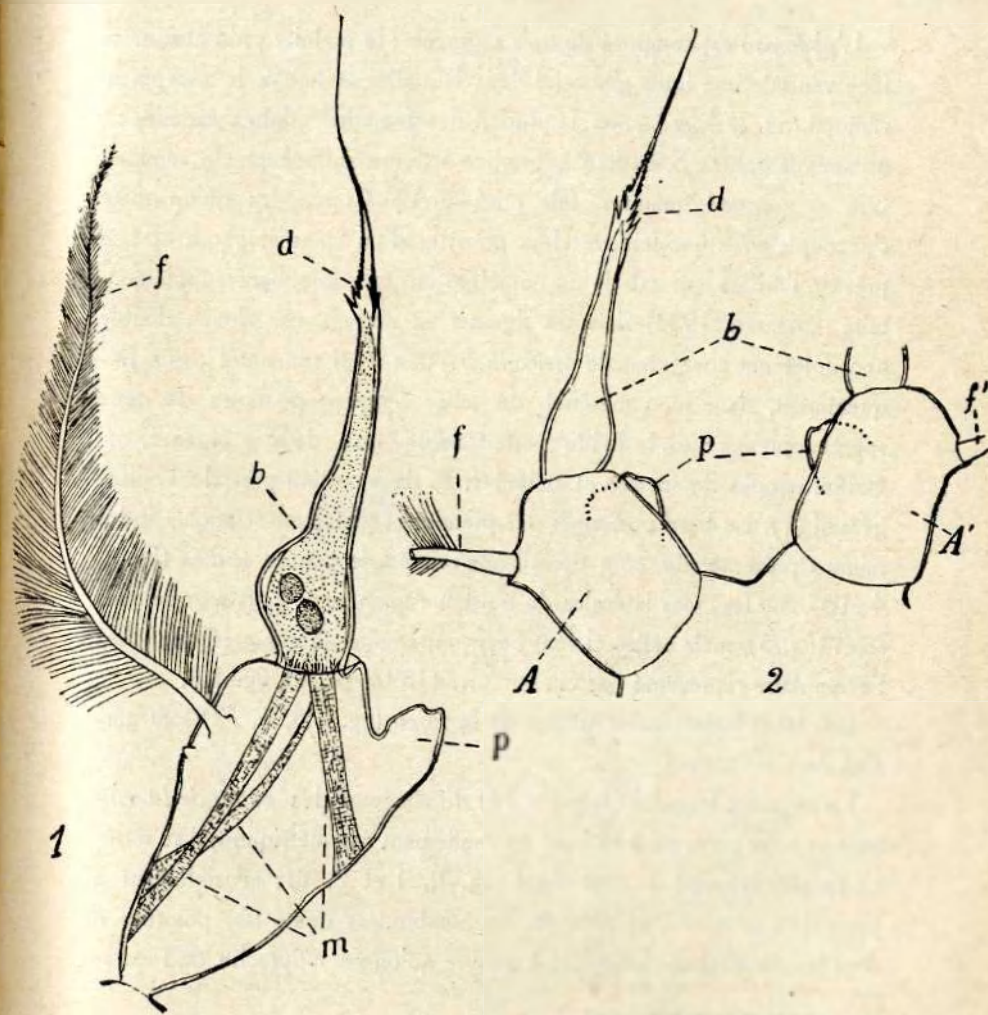
Fig. II. — Acartia tonsa DANA (♀ adulte).
