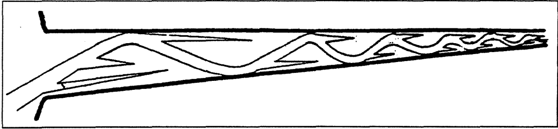
Figuur 2.5 Schema van een ideaal systeem van de Westerschelde met een ebgeul en vloedsharen (bron: Van Veen, 1950).
