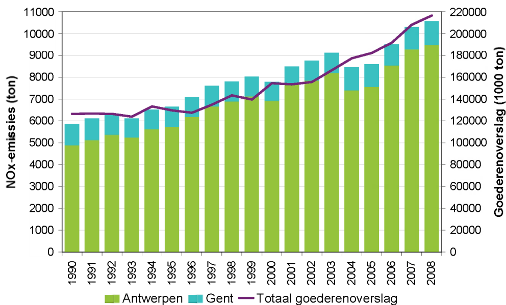
Figuur 6: Ontwikkeling in de jaarlijkse uitstoot van NO x door de scheepvaart van, naar en in GHA en Havenbedrijf Gent (1990-2008). Bron: EMMOSS model; TML in opdracht van VMM. Gegevens goederenoverslag Vlaamse Havencommissie [14].
