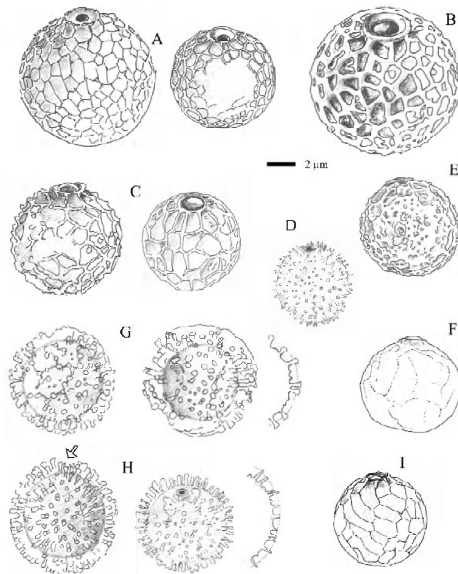
Fig. 5. a. Archaeomonas cf. areolata Deflandre var. 1. b. A. neoreticulosa sp. nov. c. A. cf. speciosa Deflandre. d. A. cf. japonica Deflandre. e. A. auranticutosa sp. nov. f. A. cf. colligera Hajós. g. Litheusphaerella cf. spectabilis Deflandre forma 1. h. L. cf. spectabilis Deflandre forma 2 (ellipsoid specimen, arrow indicates the position of the pore system, surrounded by smaller spines). i. A. arcuata sp. nov.
