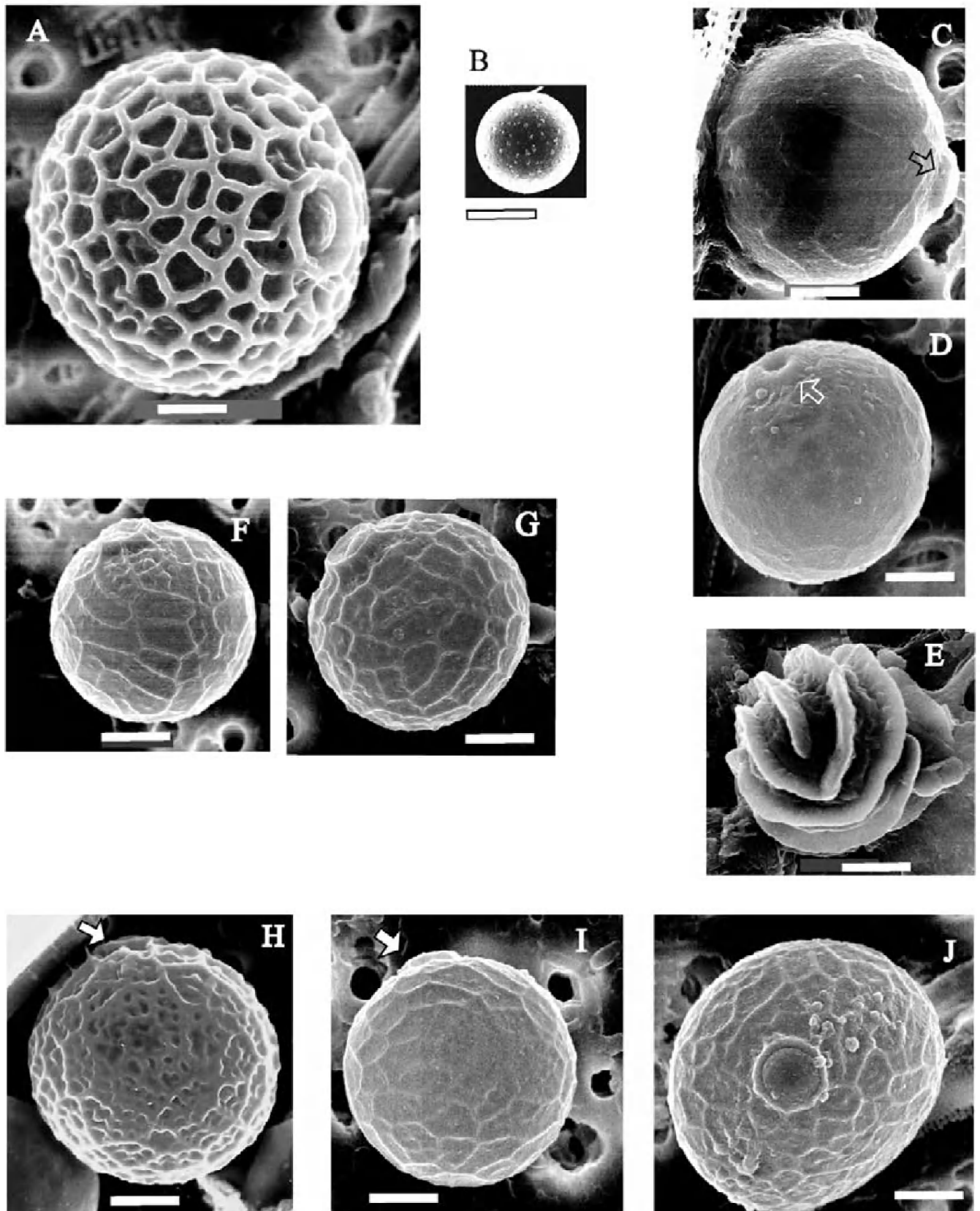
Fig. 1. a. Archaeomonas neoreticulosa sp. nov. b. (?) A. cf inconspicua Deflandre. c. & d. A. cf colligera Hajós. e. (?) A. cf heteroptera Deflandre. f. (& g?). A. arcuata sp. nov. h. (& i, j?). A. auranticutosa sp. nov. Scale bars = 2 \mu m.
