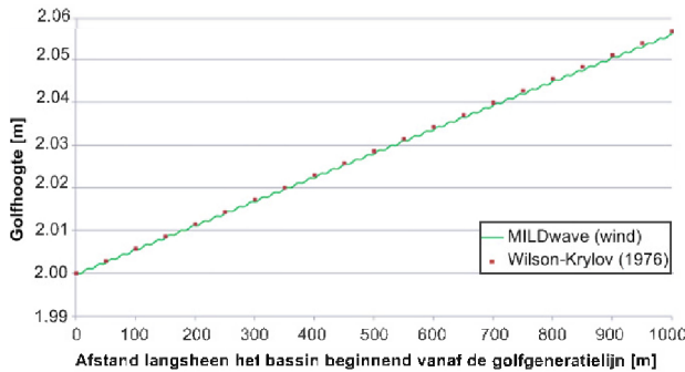
Fig. 1. Testcase 4-6: Groei van de golfhoogte Hs langs een longitudinale sectie van het numeriek bassin: MILDwave resultaten (volle lijn), Wilson-Krylov groeicurve (puntlijn).
