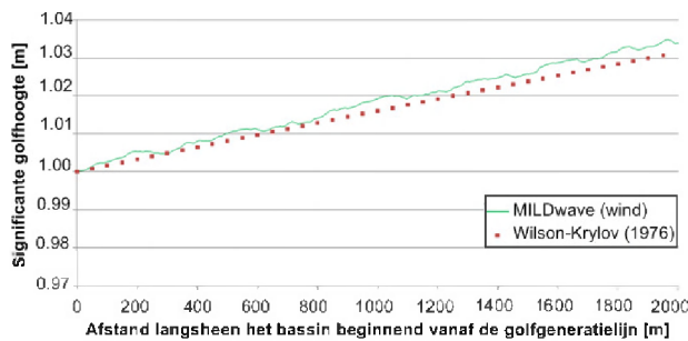
Fig. 2. Testcase J-4: Groei van de golfhoogte Hs langs een longitudinale sectie van het numeriek bassin: MILDwave resultaten (volle lijn), Wilson-Krylov groeicurve (puntlijn).
