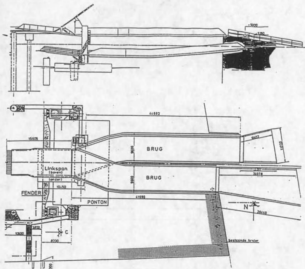
DE NIEUWE ONT- EN INSCHEPINGSBRUG GEBOUWD IN IN 1991 t.b.v. JUMBO-FERRIES, (Brug 4).
