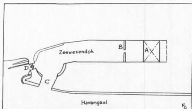
Fig. nr. 21. Inplanting "Schiffsbunker". A: snelbootbunker. B: vlottend scherm. C: nieuwe toegangsgul. D: brug geworpen over de sluis.
