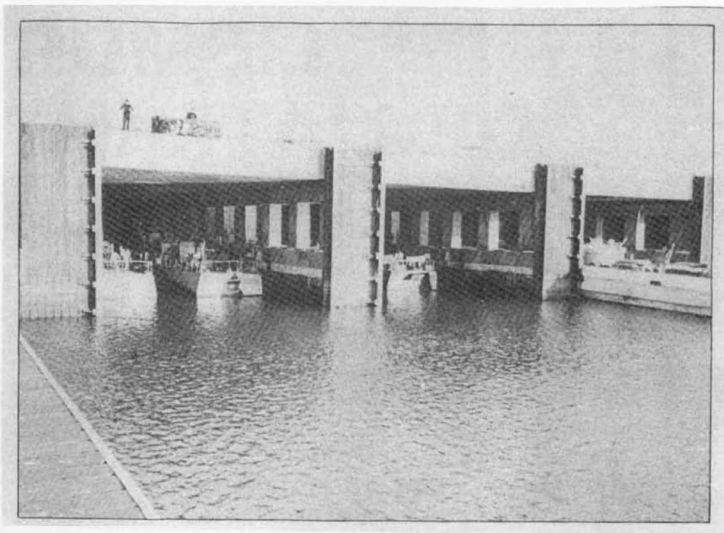
Fig. nr. 23. Haven Oostende, 1943. Zicht op de snelbotenbunker in het Zeewezendok. Bemerk de vier S-boote afgemeerd in de bunker, veilig voor alle luchtaanvallen en beschietingen vanuit zee.
