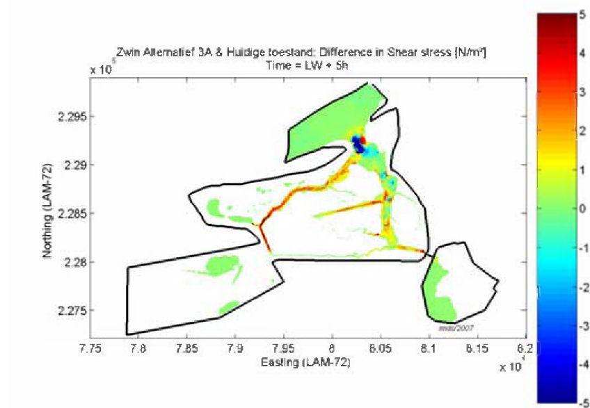
Figuur 48: Verschil in schuifspanning tussen de huidige toestand en alternatief 3A, 5 uur na laag water
