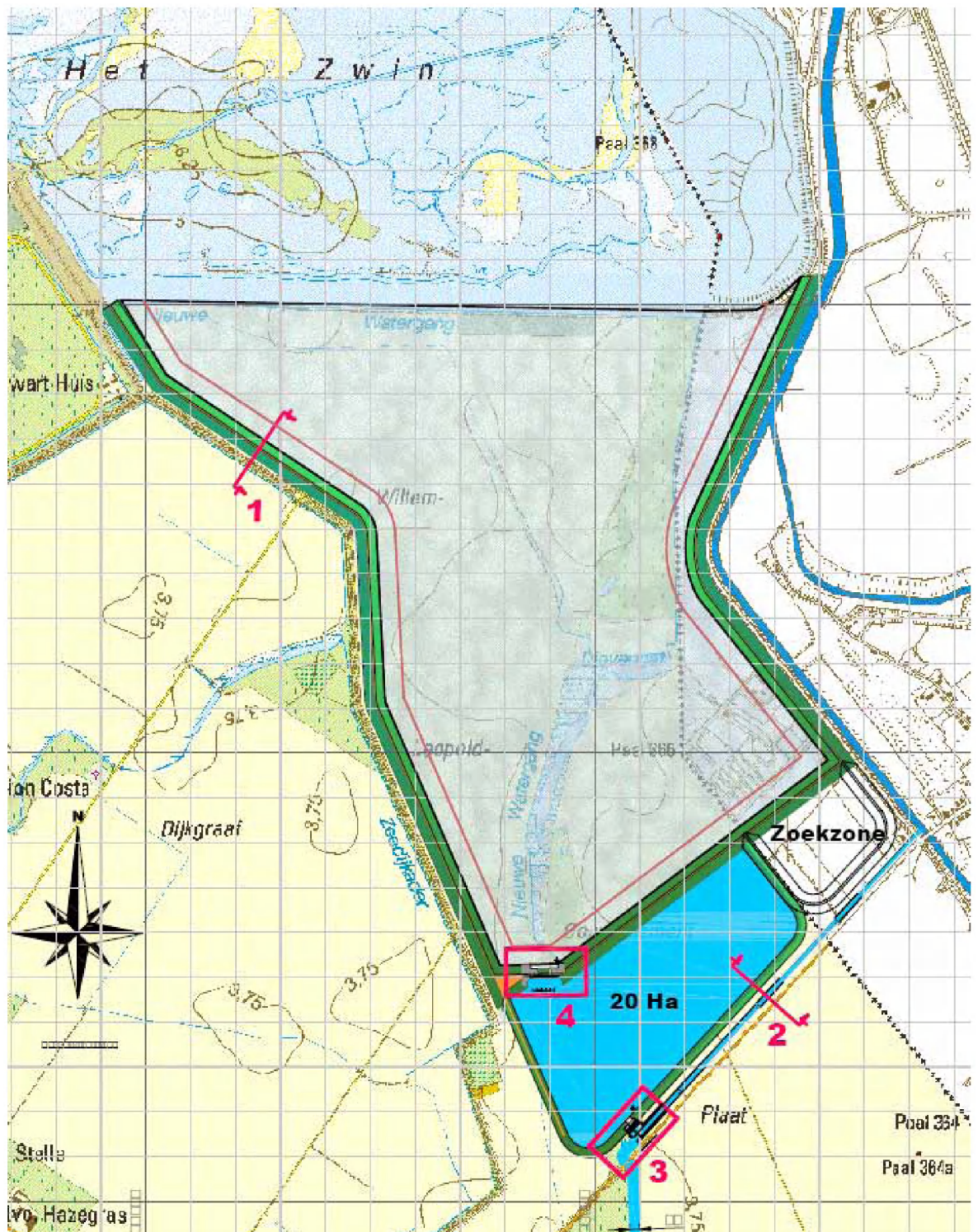
Figuur 37: Alternatief 2B met spuirom (voorontwerp)
