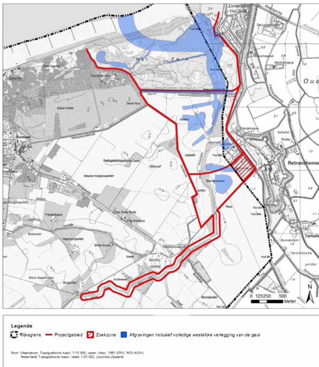
Figuur 29: Situering van de westwaarts verlegde Zwingeul
