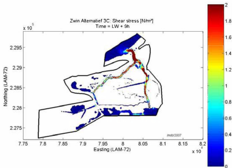
Figuur 63: Schuifspanning voor alternatief 3C, 9 uur na laag water
