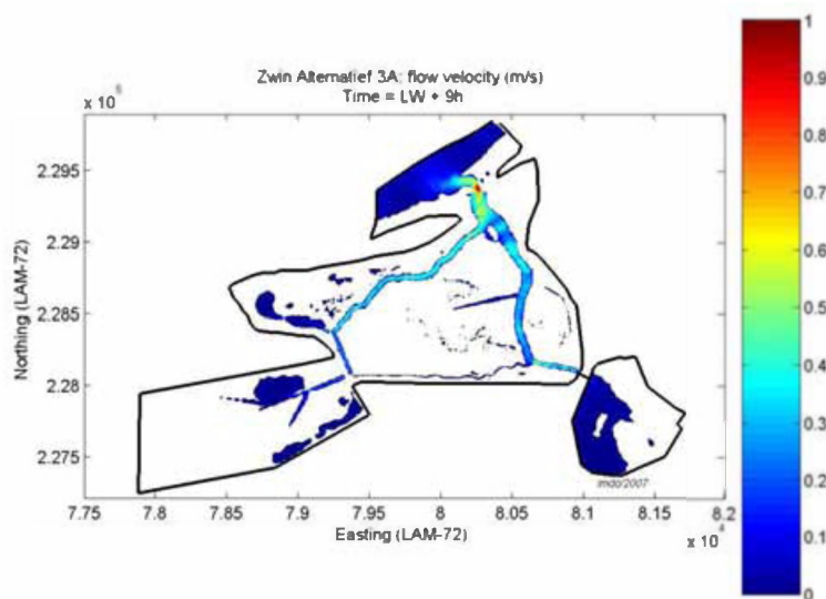
Figuur 47: Maximale stroomsnelheid bij uitstroom voor alternatief 3A
