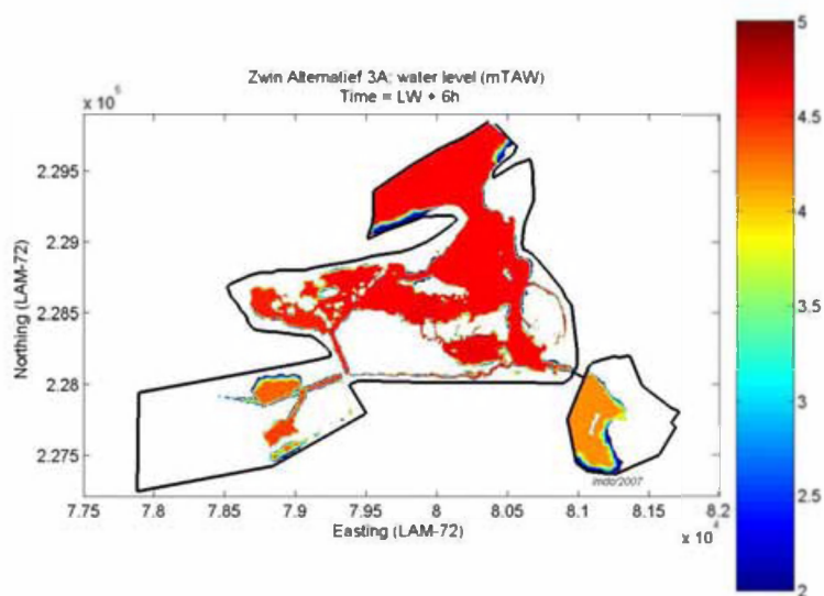
Figuur 54: Waterstand in het volledige gebied, voor het alternatief 3A op 6 h na LW
