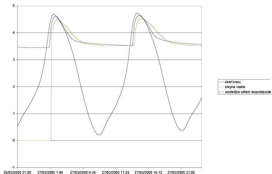
Figuur 56: Waterstand in de geulen voor de Kleynse Vlakte en de Oostelijke Willem Leopoldpolder
