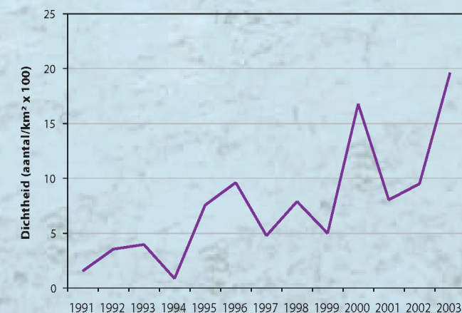
Figuur 5.17 Voorkomen bruinvissen (dichtheid) op de Noordzee, Nederlands Continentaal Plat.
