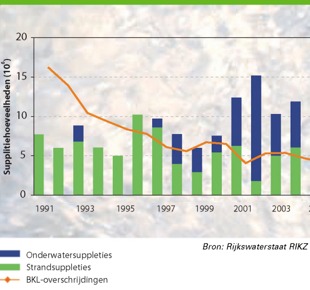
Figuur 3.2 Jaarlijkse suppletiehoeveelheden en percentages raaien waarin de Basiskustlijn is overschreden.
