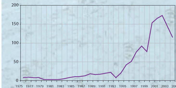
Figuur 5.19 Gewone zeehond in het deltagebied, maximum aantal per jaar
