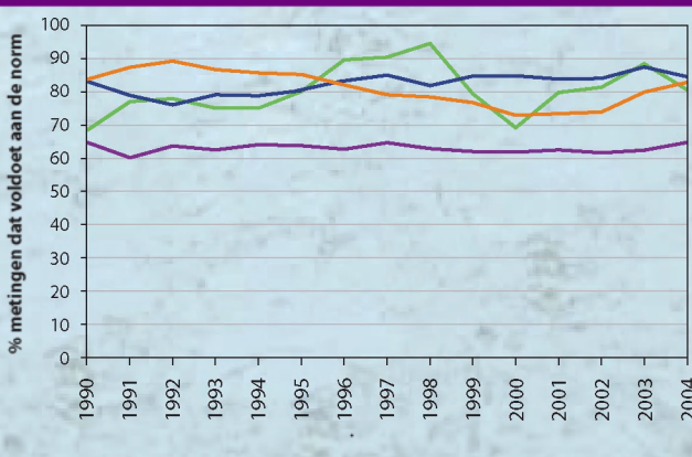
Figuur 5.8 Zware metalen in oppervlaktewater.
