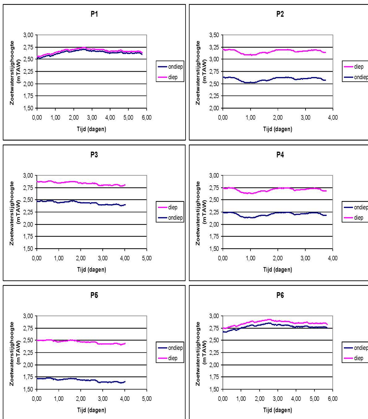
Figuur 4.1 Zoetwaterstijghoogten in mTAW in de observatieputten in het studiegebied.
