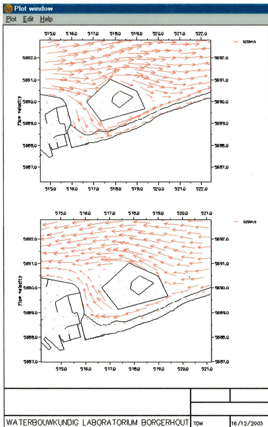
Figuur 8 : Stromingspatroon bij maximum vloodsnelheid (boven) en maximum ebsnelheid (onder) voor toestand Tv
