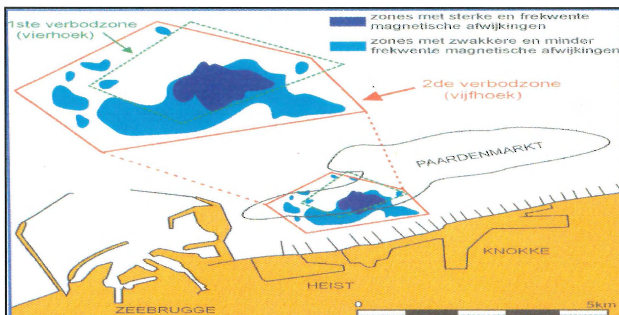
Figuur 3. Resultaten van magnetisch onderzoek uitgevoerd in 1989. De donkerblauwe zone wordt beschouwd als kerngebied. Bron: OSTC, 2002. Scientific Support Plan for a Sustainable Development Policy Paardenmarkt Site Evaluation.
