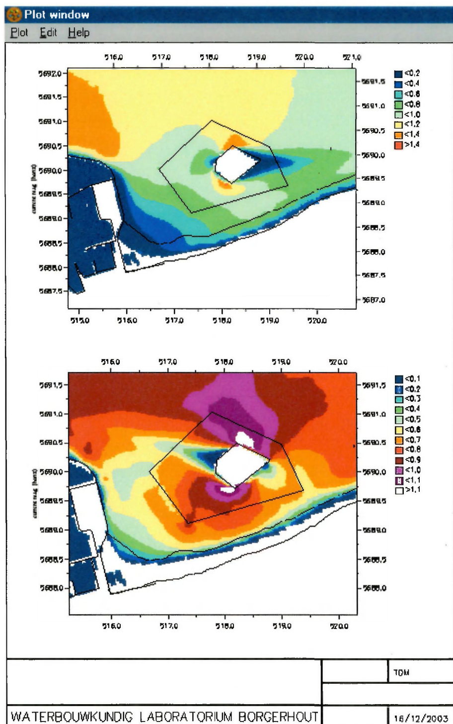
Figuur 11 : Snelheidsgroottes (m/s) bij maximum vloodsnelheid (boven) en maximum ebsnelheid (onder) voor toestand Tg
