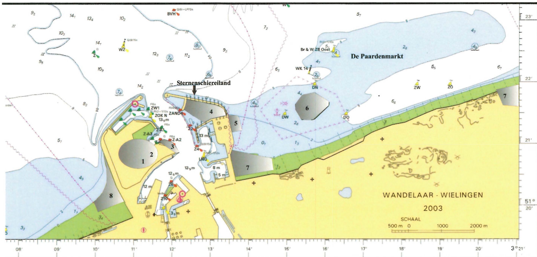
Figuur 1 Locatie van de verschillende alternatieven. 1. Ongeslacht maken huidige broedterreinen. 2. Huidige situatie handhaven. 3. Inrichten kleine gebieden. 4. Uitbreiding van het huidige sternenschiereiland. 5. Schiereiland oostelijke havendam. 6. Eiland voor de kust. 7. Geschikt maken bestaande natuurgebieden. 8. Strandvlakte Zeebrugge Bad.
