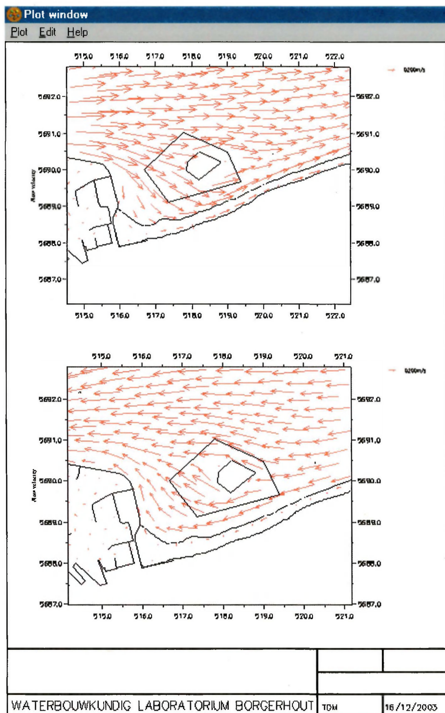
Figuur 7 : Stromingspatroon bij maximum vloedsnelheid (boven) en maximum ebsnelheid (onder) voor toestand Tg
