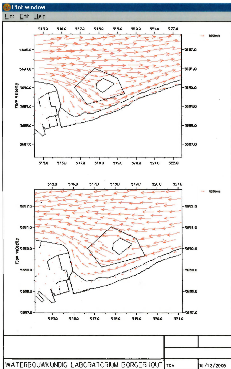
Figuur 6 : Stromingspatroon bij maximum vloodsnelheid (boven) en maximum ebsnelheid (onder) voor toestand Tf
