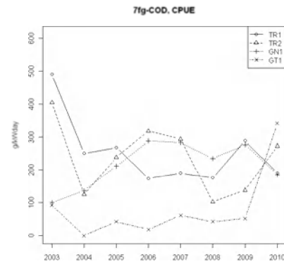
CPUE 7 fg
