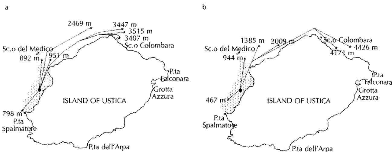
Figure 1 - Homing of dusky grouper following release in the core area of the marine reserve in (a): 25 November 1997 (group 1) and (b): 30 October - 6 November 1998 (group 2). The straight lines represent the shortest distances (given next to site of capture) between the site of release (•) and the sites of capture (*). The stippled area represents the core area of the marine reserve. / Retour au gîte des mérour noirs après le lâcher dans l'aire centrale de la réserve marine (a) : le 25 novembre 1997 (groupe 1) et (b) : le 30 octobre - 6 novembre 1998 (groupe 2). Les lignes droites représentent les distances les plus courtes (indiquées près du site de capture) entre le site de lâcher (•) et les sites de capture (*). La zone ombrée représente la réserve intégrale.
