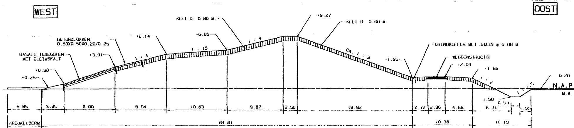
DWARSPROFIEL 1 (BESTAANDE SITUATIE INCL. OVERHOOGTE)
