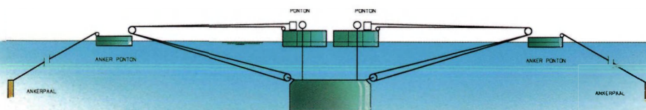
AFZINKSYSTEEM TUNNELEMENT
