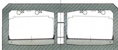
DWARSPROFIEL TUNNELEMENT
