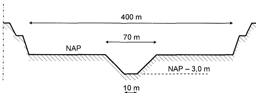
Figuur 5.8. Schematisch doorstroomprofiel bres (verschaald)
