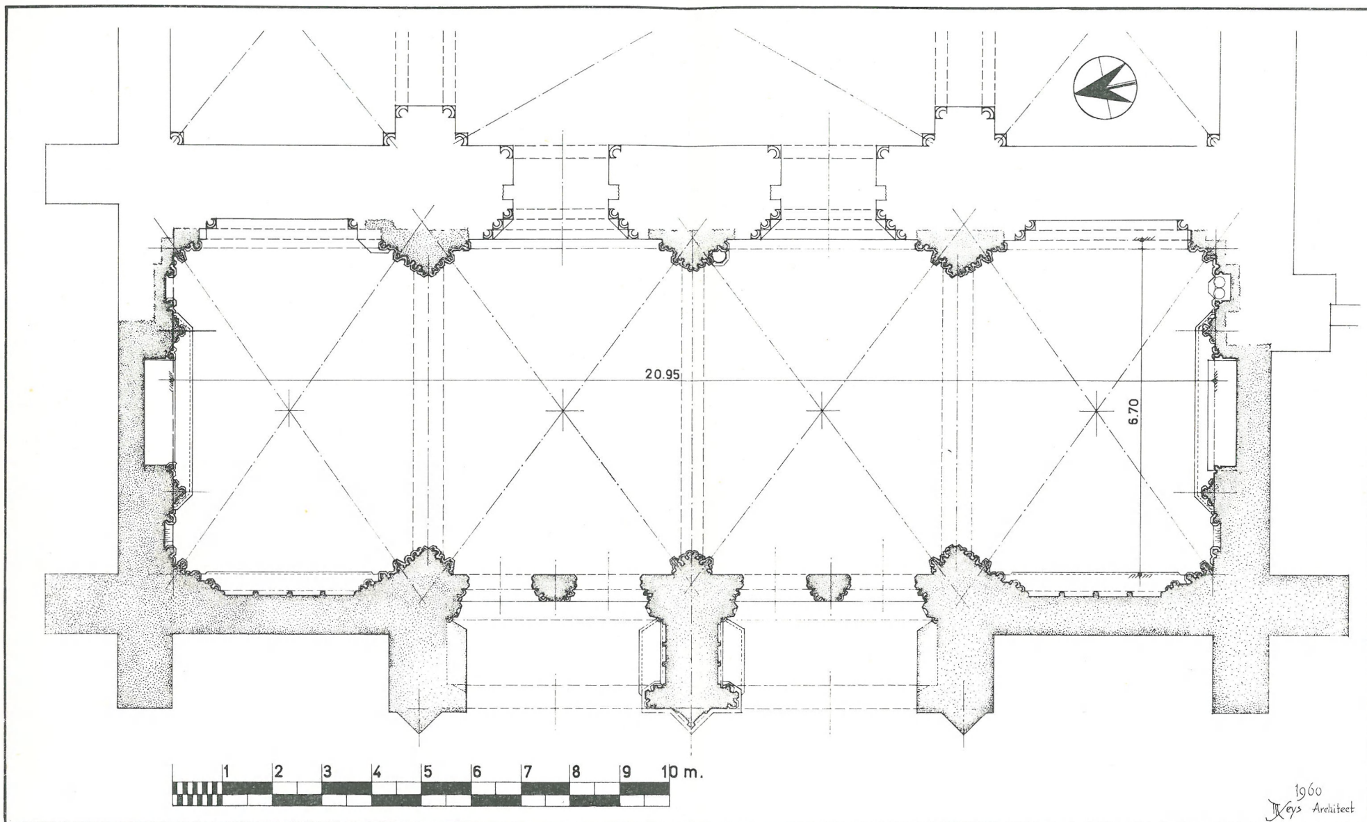
Abdijkerk Ten Duinen. Grondplan van westmuur en voorportaal (peil onder de vensters).
