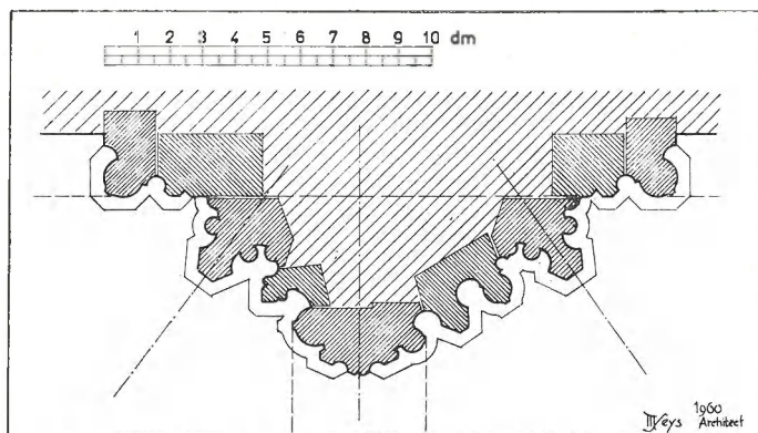
Voorpoortaal, doorsnede over de oostelijke pijlerbundel onder de zuidelijke moerboog. Eerste helft 14e eeuw.
