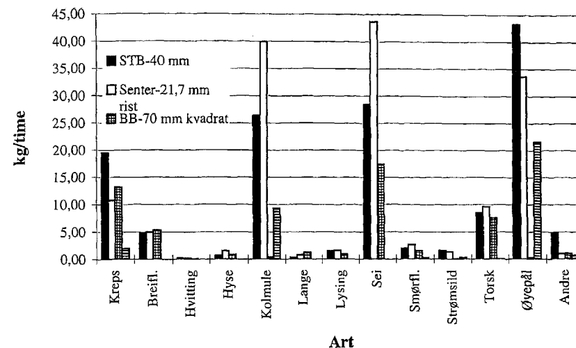
Figur 13. Gjennomsnittsfangster i trippeltrålen fra forsøkene på Egersundbanken i 1996, riggget med 40 mm vanlig masker, 21,7 mm rist og 70 mm kvadratiske masker [Average catches (kg/hr) in the triple trawl during the experiments in 1996, rigged with 40 mm diamond meshes, 21,7 mm grid and 70 mm square meshes].
