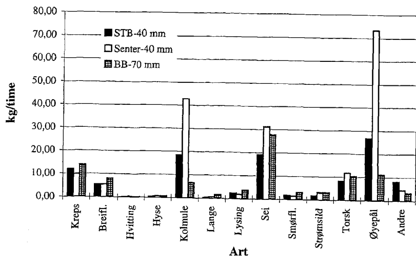
Figur 12. Gjennomsnittsfangster i trippeltrålen fra forsøkene på Egersundbanken i 1996, riggget med 40 mm og 70 mm vanlige masker [Average catches (kg/hr) in the triple trawl during the trials in 1996, rigged with 40 and 70 mm diamond meshes].
