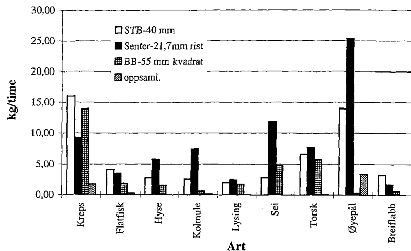
Figur 11. Gjennomsnittsfangster i trippeltrålen for forsøkene i Skagerrak i 1995, riggget med 40 mm vanlige masker, 21,7 mm rist og 55 mm kvadratiske masker [Average catches in the triple trawl during the trials in 1995, rigged with 40 mm diamond meshes, 21,7 mm grid and 55 mm square meshes].
