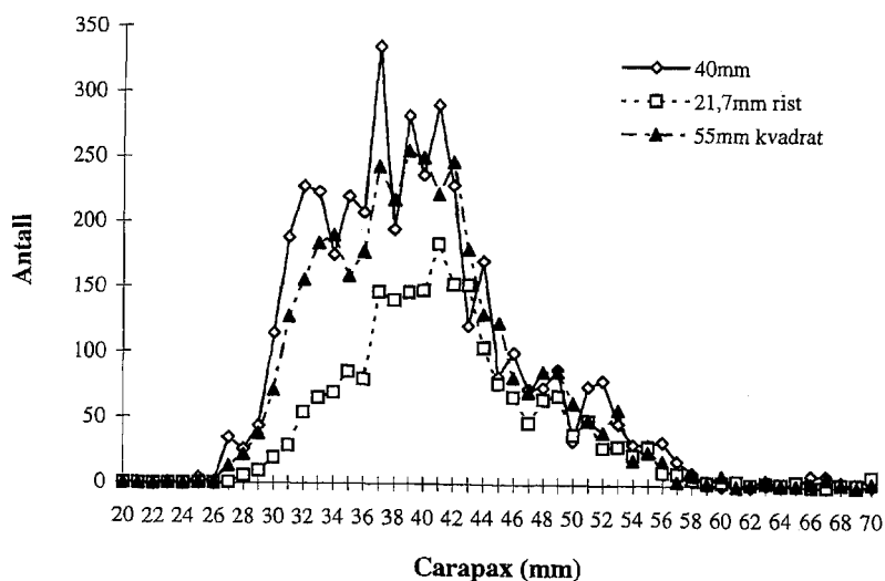
Figur 18. Lengdefordeling av sjøkreps fanget i trippeltrål fra forsøkene på Egersundbanken i 1995, rigget med 40 mm vanlige masker, 21,7 mm rist og 55 mm kvadratiske masker [Length distribution of Norway lobster caught in triple trawl during the experiments in 1995, rigged with 40 mm diamond meshes, 21.7 mm grid and 55 mm square meshes].
