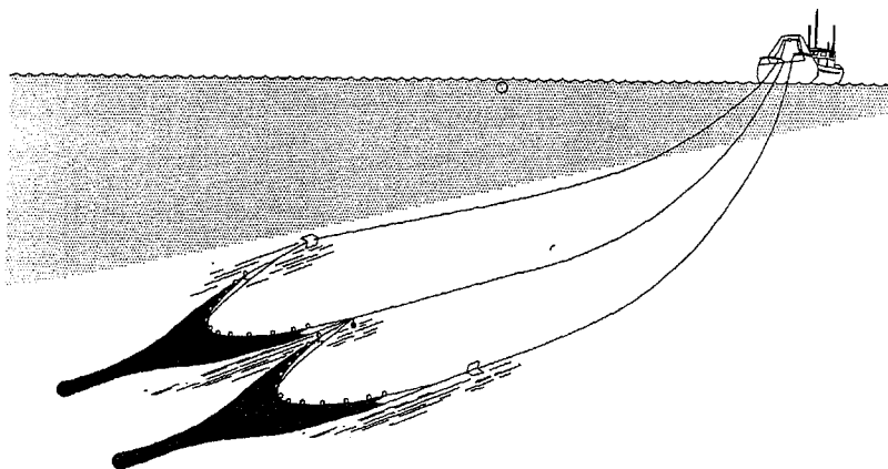
Figur 1a. Tvillingtrål rigget med tre trålwirer [Twin trawl rigged with three towing warps].
