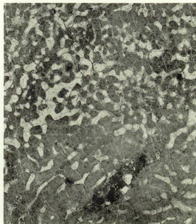
Fig. 4. - Trupetostroma crassum nov. sp.
