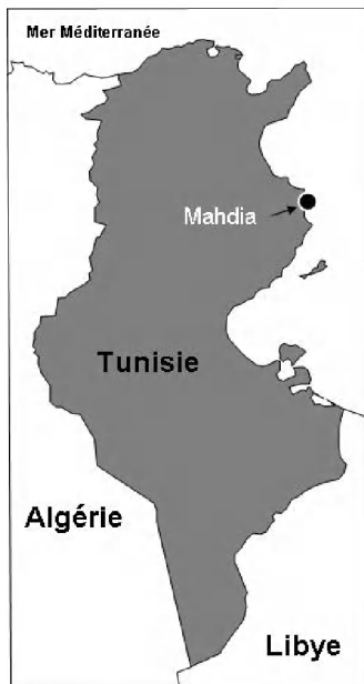
Carte 1
