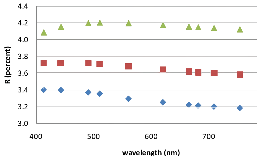
AOT=0.3, SZA=29°
