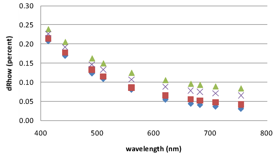
SZA=59°, ws=1 m/s, AOT=0.3
