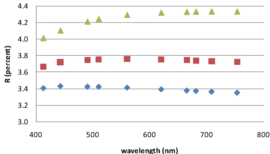
AOT=0.3, SZA=59°
