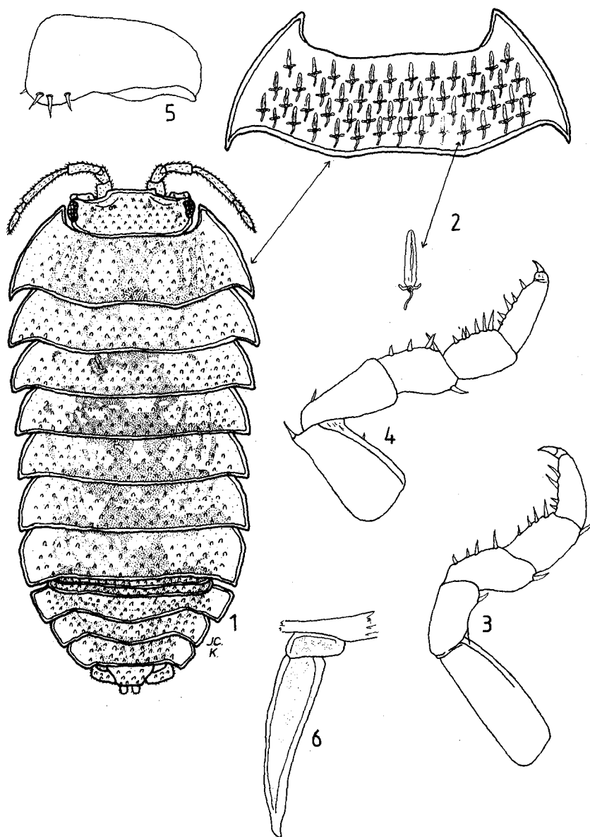
Fig. 1-6: Armadillidium album DOLLFUS, 1889. - 1: vue dorsale; 2: premier périonite avec soies écaillés; 3: premier péréopode mâle; 4: septième péréopode mâle; 5: exopodite du premier pléopode; 6: endopodite du premier pléopode mâle.
