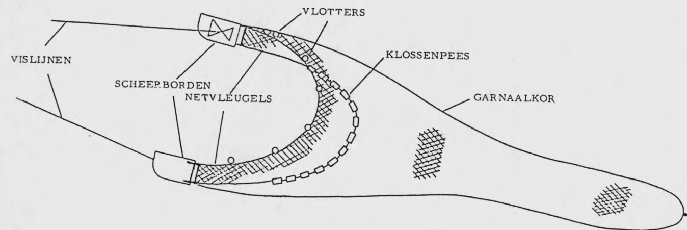
Figuur 3 - Schematische voorstelling van de optuiging van een garnaalbordennet.
