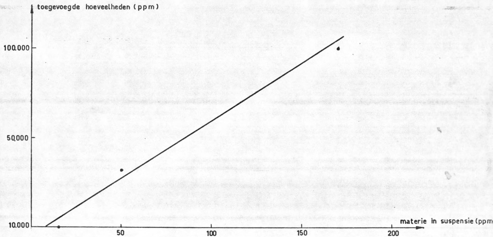
Fig. 3 - Relatieve pollutant concentraties, toegevoegd en in suspensie
