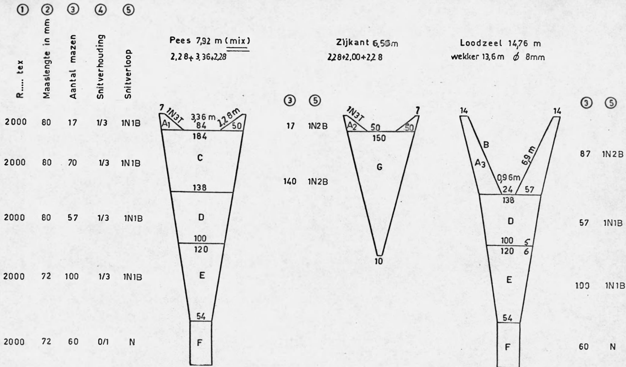
Figuur 1 - Plan van het semi_pelagisch net (Systeem 1) .
