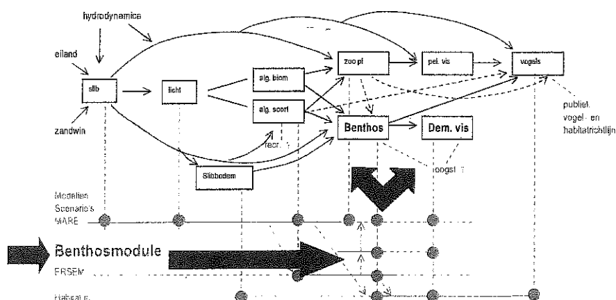
Afbeelding 1. Positie van het benthosmodel in de effectenketen Noordzee
