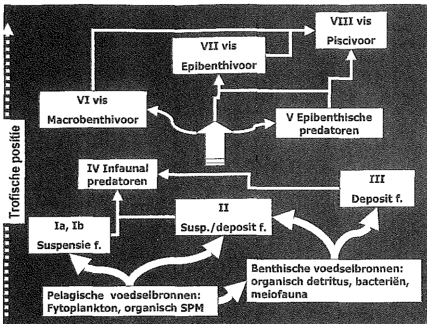
Afbeelding 4. Voedselweb in het BENBOX-model. De groepen Ia, Ib (suspension feeders) worden voornamelijk direct door pelagische voedselbronnen aangestuurd (fytoplankton concentratie) terwijl de groep III (deposit feeders) voornamelijk op benthische voedselbronnen foerageert. Groep II (interface feeders, surface deposit feeders) zit daartussen in. Groep IV (infaunal predators) foerageert op de groepen I-III. Groepen V-VIII (epibenthos en vis) hebben een hoger trofische positie en foerageren op onderliggende groepen maar ook op kleinere vertegenwoordigers uit de dezelfde groep. Deze relaties zijn niet allemaal met pijlen aangegeven. Voorbeeldsoorten uit verschillende groepen zijn in 2.4 beschrijven.
