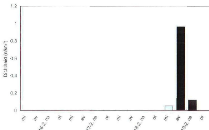
Figuur 27 2D-Dichtheid (echo's/km²) boven 100 meter in februari 1999. De dichtheden zijn gebaseerd op de verticale scan (kijkrichting 284°) en gesplitst naar nacht, ochtend, middag en avond. Wanneer de trek uit of naar zee is waargenomen zijn tevens de dichtheden van de verticale scan, kijkrichting 194°, door een • weergegeven. Alleen dagdelen met één dominante, significante vliegrichting zijn weergegeven. 2D-density (echoes per km²) above 100m altitude in February 1999. Densities are based on the vertical scan towards 284° and grouped by night, morning, noon and evening. When bird movements from or towards the sea were observed, the results of the vertical scan towards 194° are also presented and marked with a •. Only day parts with a unimodal distribution and a significant mean flight direction are presented.
