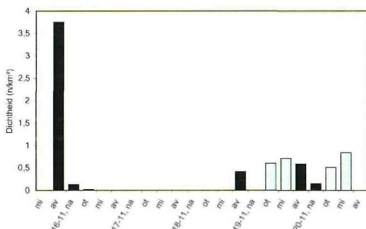
Figuur 48 2D-Dichtheid (echo's/km²) boven 100 meter in november 1999. De dichtheden zijn gebaseerd op de verticale scan (kijkrichting 284°) en gesplitst naar nacht, ochtend, middag en avond. Wanneer de trek uit of naar zee is waargenomen zijn tevens de dichtheden van de verticale scan, kijkrichting 194°, door een • weergegeven. Alleen dagdelen met één dominante, significante vliegrichting zijn weergegeven. 2D-density (echoes per km²) above 100m altitude in November 1999. Densities are based on the vertical scan towards 284° and divided by night, morning, noon and evening. When bird movements from or towards the sea were observed, the results of the vertical scan towards 194° are also given. Only day parts with a unimodal distribution and a significant mean flight direction are presented.
