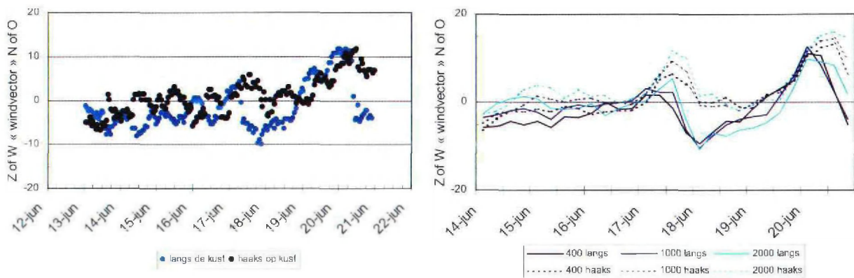
Figuur 35 Windvectoren (m/s) ten opzichte van trek langs respectievelijk haaks op de kust, juni 1999, IJmuiden. In de linker figuur zijn de windvectoren afgeleid uit de gemeten wind op 10 meter hoogte. In de rechter figuur wordt de windvector op 400, 1000 en 2000 meter hoogte uit het HIRLAM model weergegeven, langs (doorgetrokken lijn) of haaks op (gestippelde lijn) de kustlijn. Wind vectors related to bird movements along (light blue or line) and perpendicular to (dark blue or dashed line) the coastline, June 1999. Left figure: measured wind vectors at 10 m altitude. Right figure: wind vectors at 400, 1000 and 2000 m altitude, obtained from HIRLAM model.
