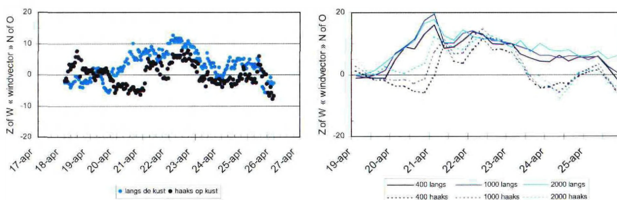
Figuur 31 Windvectoren (m/s) ten opzichte van trek langs respectievelijk haaks op de kust, april 1999, IJmuiden. In de linker figuur zijn de windvectoren afgeleid uit de gemeten wind op 10 meter hoogte. In de rechter figuur wordt de windvector op 400, 1000 en 2000 meter hoogte uit het HIRLAM model weergegeven, langs (doorgetrokken lijn) of haaks op (gestippelde lijn) de kustlijn. Wind vectors related to bird movements along (light blue or line) and perpendicular to (dark blue or dashed line) the coastline, April 1999. Left figure: measured wind vectors at 10 m altitude. Right figure: wind vectors at 400, 1000 and 2000 m altitude, obtained from HIRLAM model.
