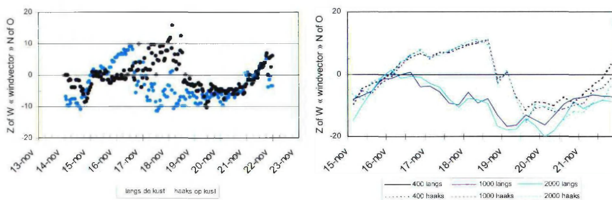
Figuur 47 Windvectors (m/s) geprojecteerd langs en haaks op de kust, november 1999, IJmuiden. In de linker figuur zijn de windvectors afgeleid uit de gemeten wind op 10 meter hoogte. In de rechter figuur wordt de windvector op 400, 1000 en 2000 meter hoogte uit het HIRLAM model weergegeven, langs (doorgetrokken lijn) of haaks op (gestippelde lijn) de kustlijn. Wind vectors related to bird movements along (light blue or line) and perpendicular to (dark blue or dashed line) the coastline, November 1999. Left figure: measured wind vectors at 10 m altitude. Right figure: wind vectors at 400, 1000 and 2000 m altitude, obtained from HIRLAM model.
