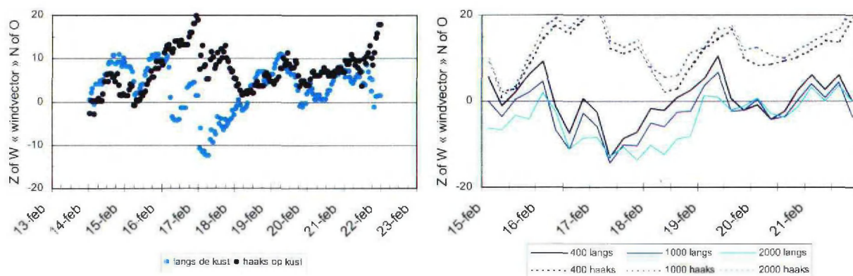
Figuur 26 Windvectors (m/s) ten opzichte van trek langs respectievelijk haaks op de kust, februari 1999, IJmuiden. In de linker figuur zijn de windvectors afgeleid uit de gemeten wind op 10 meter hoogte. In de rechter figuur wordt de windvector op 400, 1000 en 2000 meter hoogte uit het HIRLAM model weergegeven, langs (doorgetrokken lijn) of haaks op (gestippelde lijn) de kustlijn. Wind vectors related to bird movements along (light blue or line) and perpendicular to (dark blue or dashed line) the coastline, February 1999. Left figure: measured wind vectors at 10 m altitude. Right figure: wind vectors at 400, 1000 and 2000 m altitude, obtained from HIRLAM model.
