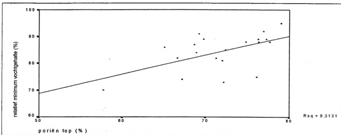
Figuur 3.34. Relatief minimum vochtgehalte i.f.v. het poriënvolume van de tophorizont.
