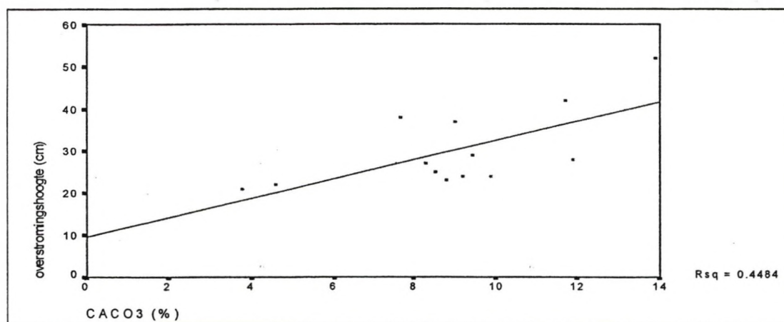
Figuur 3.28. \text{CaCO}_3 -gehalte i.f.v. overstromingshoogte.
