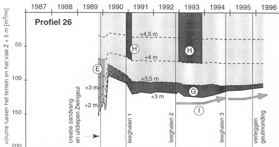
Fig. 8. Evolutie van het vrij volume tussen het terrein en het hoogtevlak van +5 m ter hoogte van profiel 26 (zuidelijke Zwingeu). Het volume werd berekend in hoogteschijven van 0,5 m. De letters worden toegelicht in de tekst.
