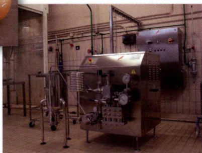
Hoge drukhomogenisator
