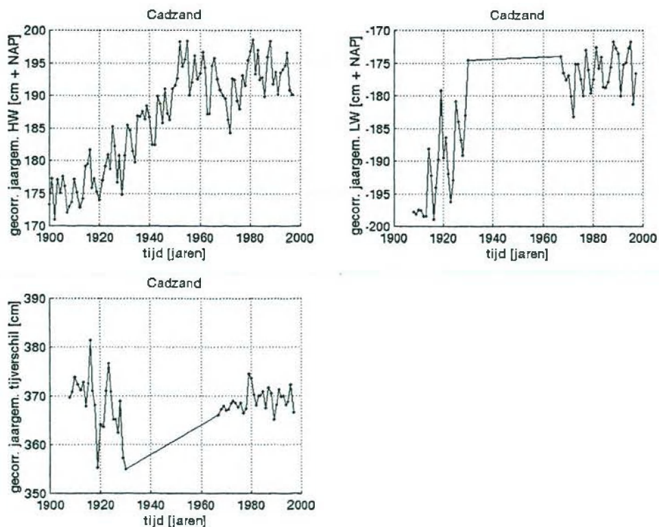
Afbeelding V.7b Gecorrigeerde tijdreeksen (Cadzand)
