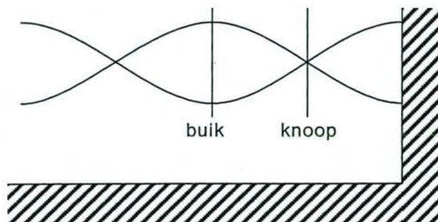
Afbeelding 7.1 Patroon staande golf in enkelzijdig gesloten bekken
