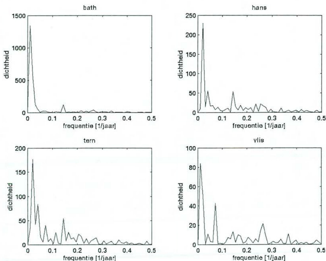
Afbeelding 5.2 Spectra van de residuen voor vier locaties
