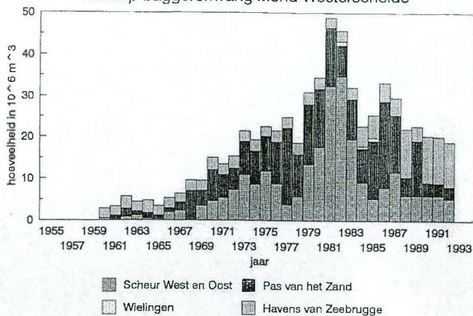
Afbeelding 4.6b. Verloop bagger- en stortomvang mond westerschelde
