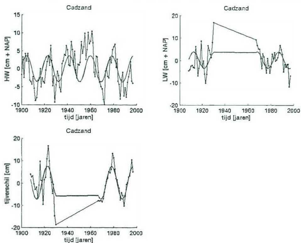
Afbeelding V.7a Tijdreeks (zonder trend) en bijpassende 18,6 jarige cyclus (Cadzand)
