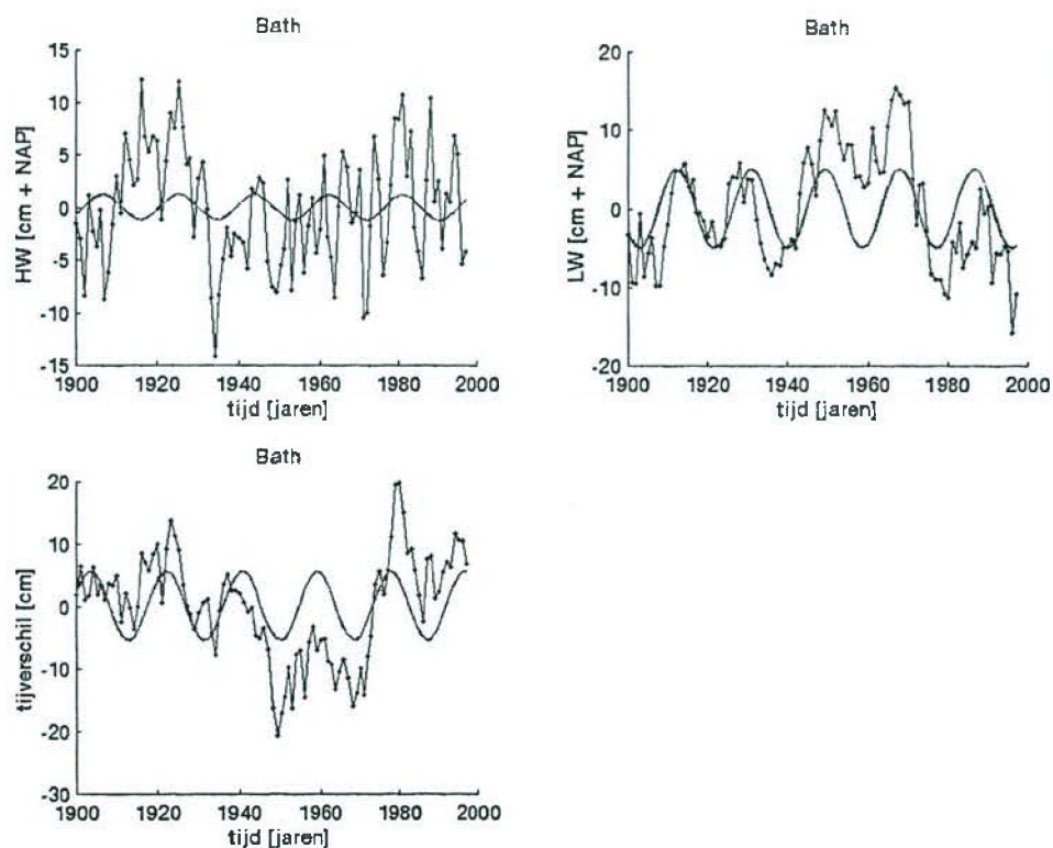
Afbeelding V.3a Tijdreeks (zonder trend) en bijpassende 18,6 jarige cyclus (Bath)
