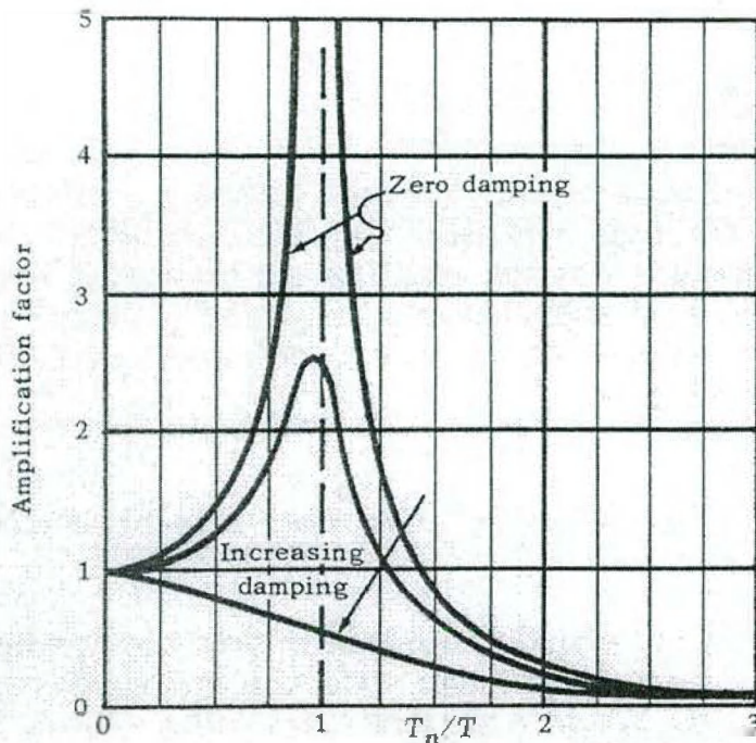
Afbeelding 7.2 Invloed wrijving op resonantie (Ippen, 1966)
