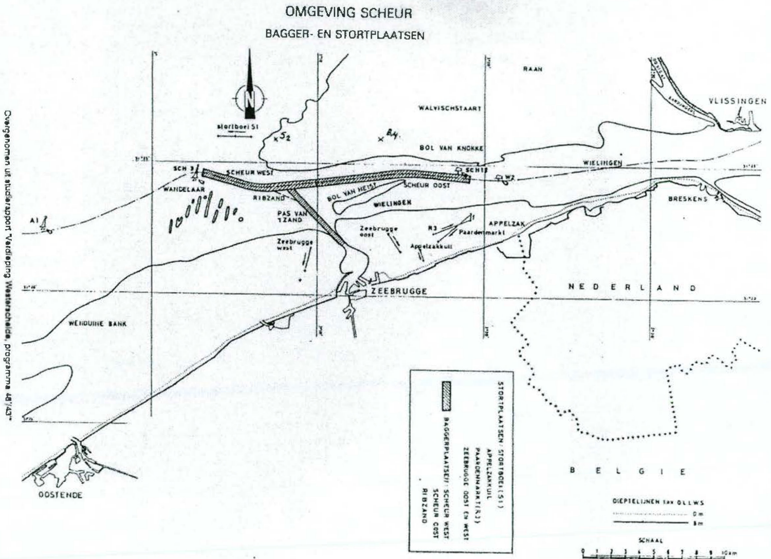
Atbeelding 4.6a. Bagger- en stortlocaties omgeving Scheur
