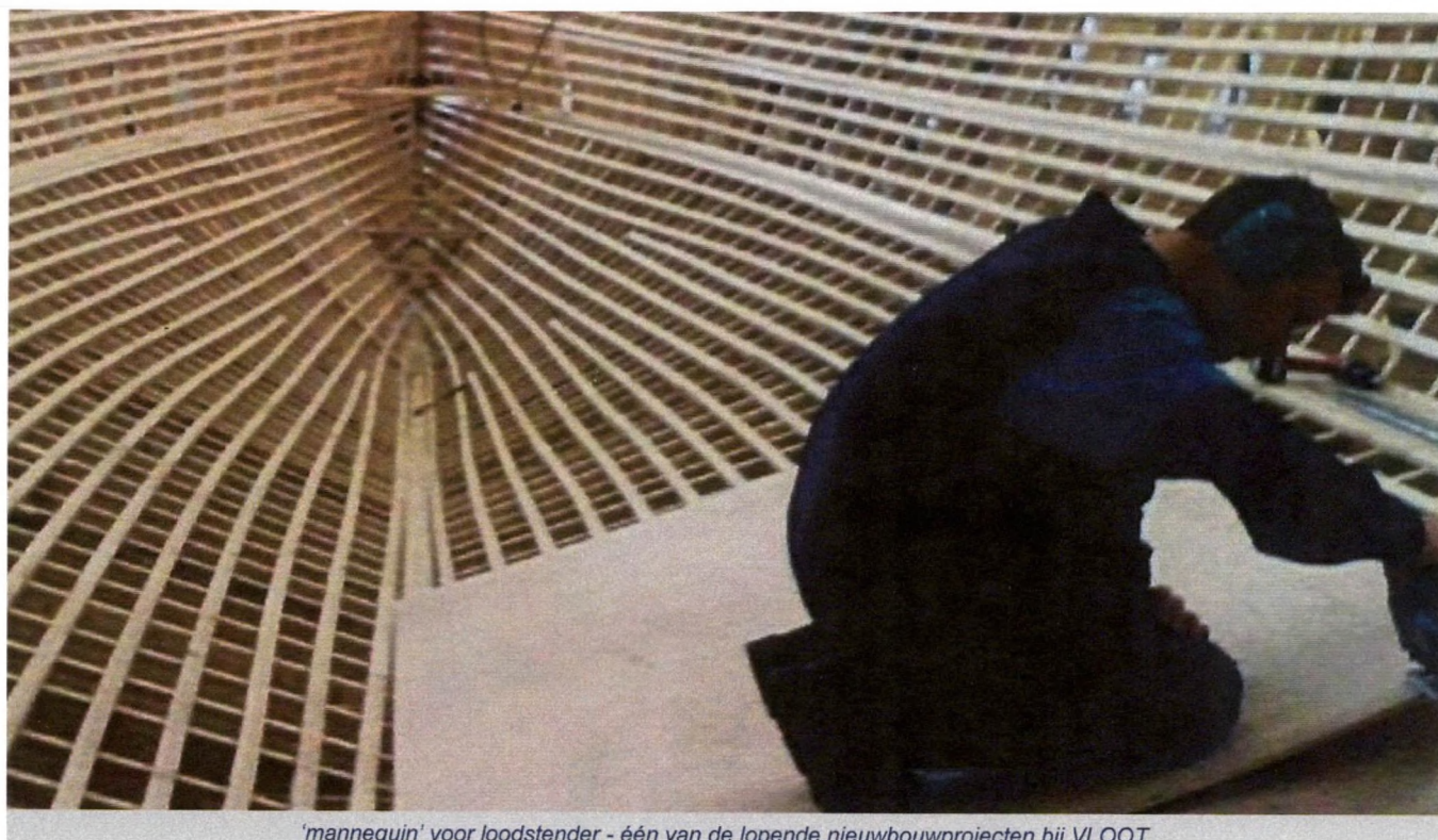
'mannequin' voor loodstender - één van de lopende nieuwbouwprojecten bij VLOOT
