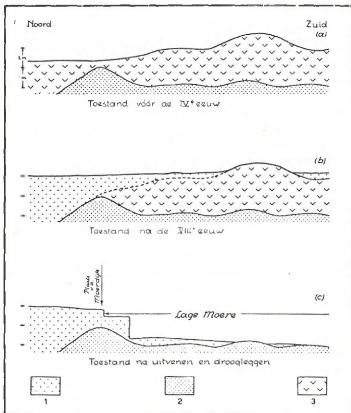
Fig. Ontstaan van de Lage Moere van Meetkerke (zonder lengteschaal).
