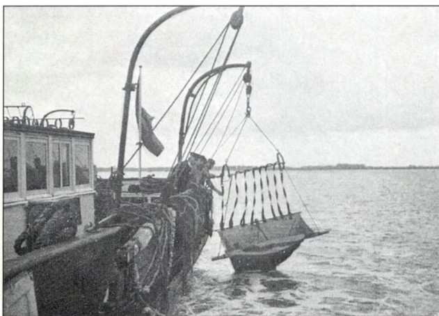
Opaling van visnet aan boord van de Sleper nr. 1 van Oostende
