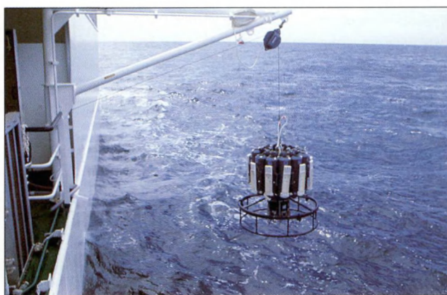
Het STD-systeem
