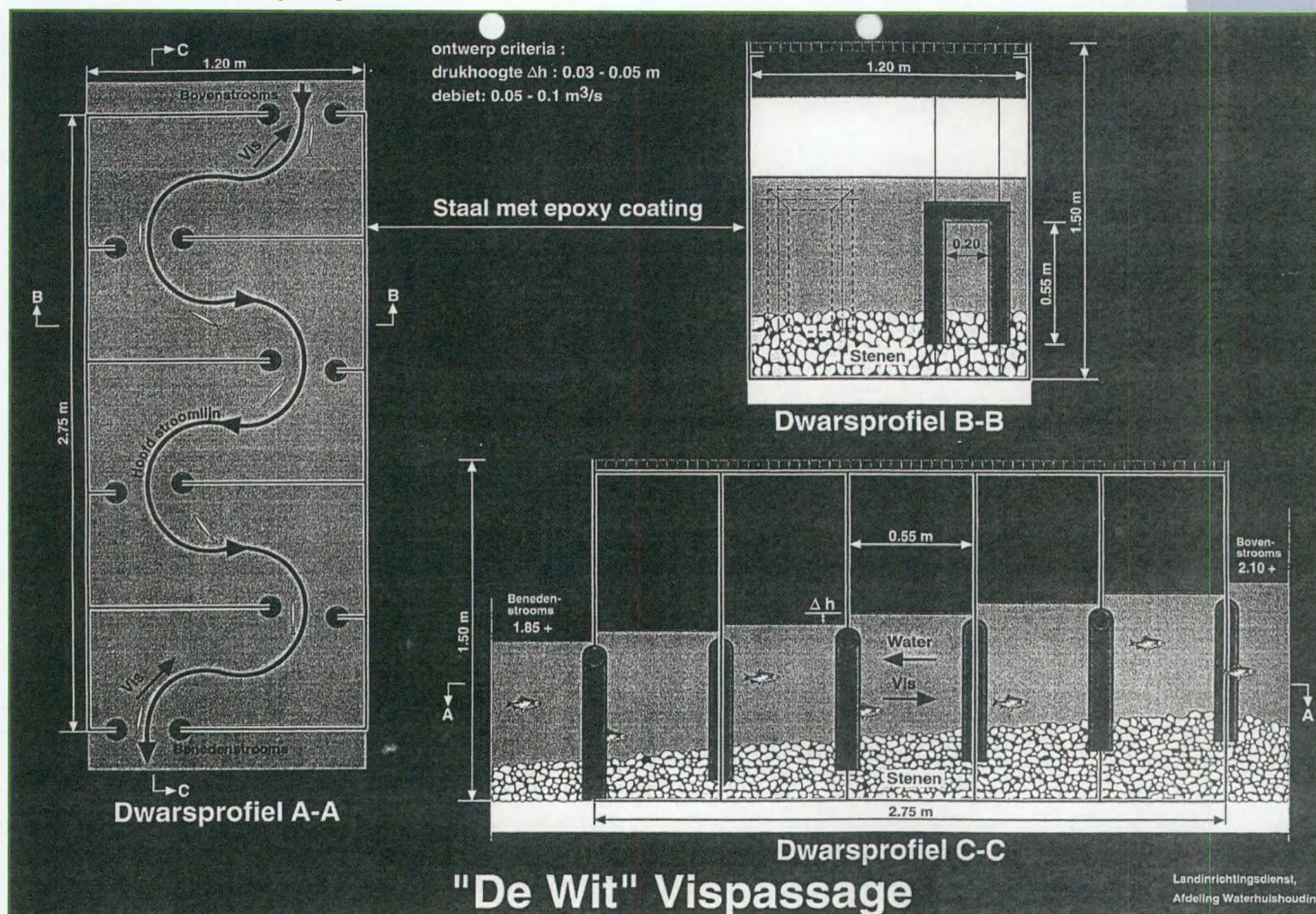
Schema van "De Wit" vispassage
