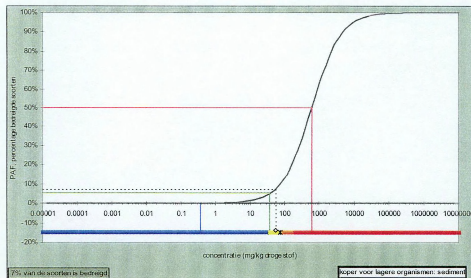
FIGUUR 18 : VERGELIJKING VAN DE KOPERCONCENTRATIE (MG/KG.DS) IN HET SEDIMENT MET DE GEVOELIGHEIDSVERDELING VOOR KOPER
