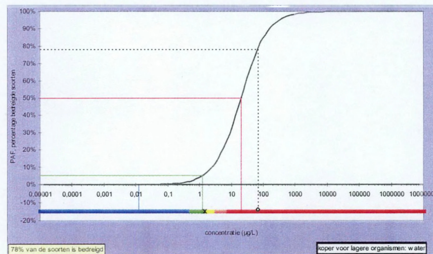
FIGUUR 17 : VERGELIJKING VAN DE GEMIDDELDE KOPERCONCENTRATIE (µg/L) IN DE WATERKOLOM MET DE GEVOELIGHEIDSVREDELING VOOR KOPER
