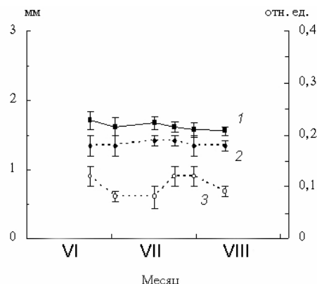
Рис. 5. Размеры эфиппийальных самок Daphnia curvirostris в течение сезона. Обозначения как на рис. 4.
