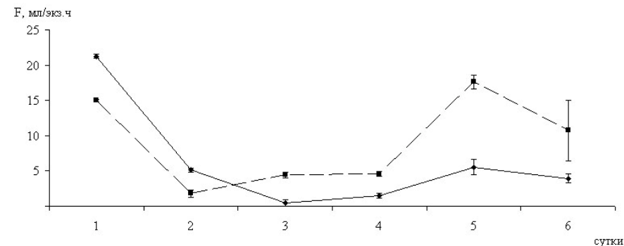
Рис. 2. Динамика скорости филътрации при низкой начальной концентрации хлореллы. Обозначения, как на рис. 1.
