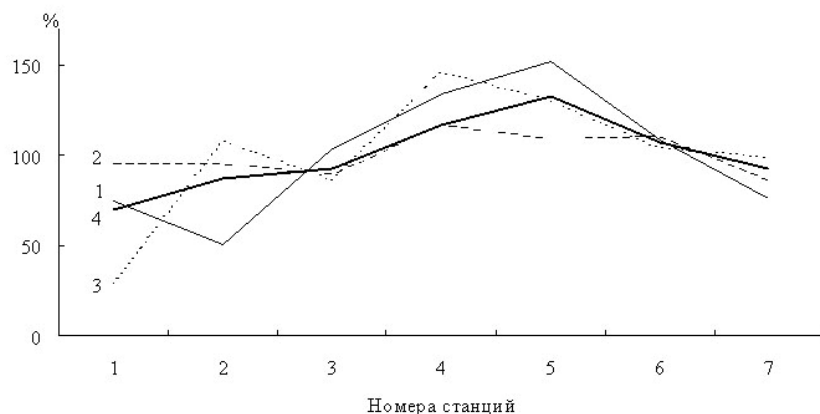
Рис. 10. Колебания значений индексов загрязнения р. Латка по зообентосу в 2003 г. по оси ординат – значения индексов, % от средней величины; по оси абсцисс – номера станций. 1 – тибифидный индекс, 2 – средняя сапробность, 3 – индекс Балушкиной, 4 – индекс КИЗ.
