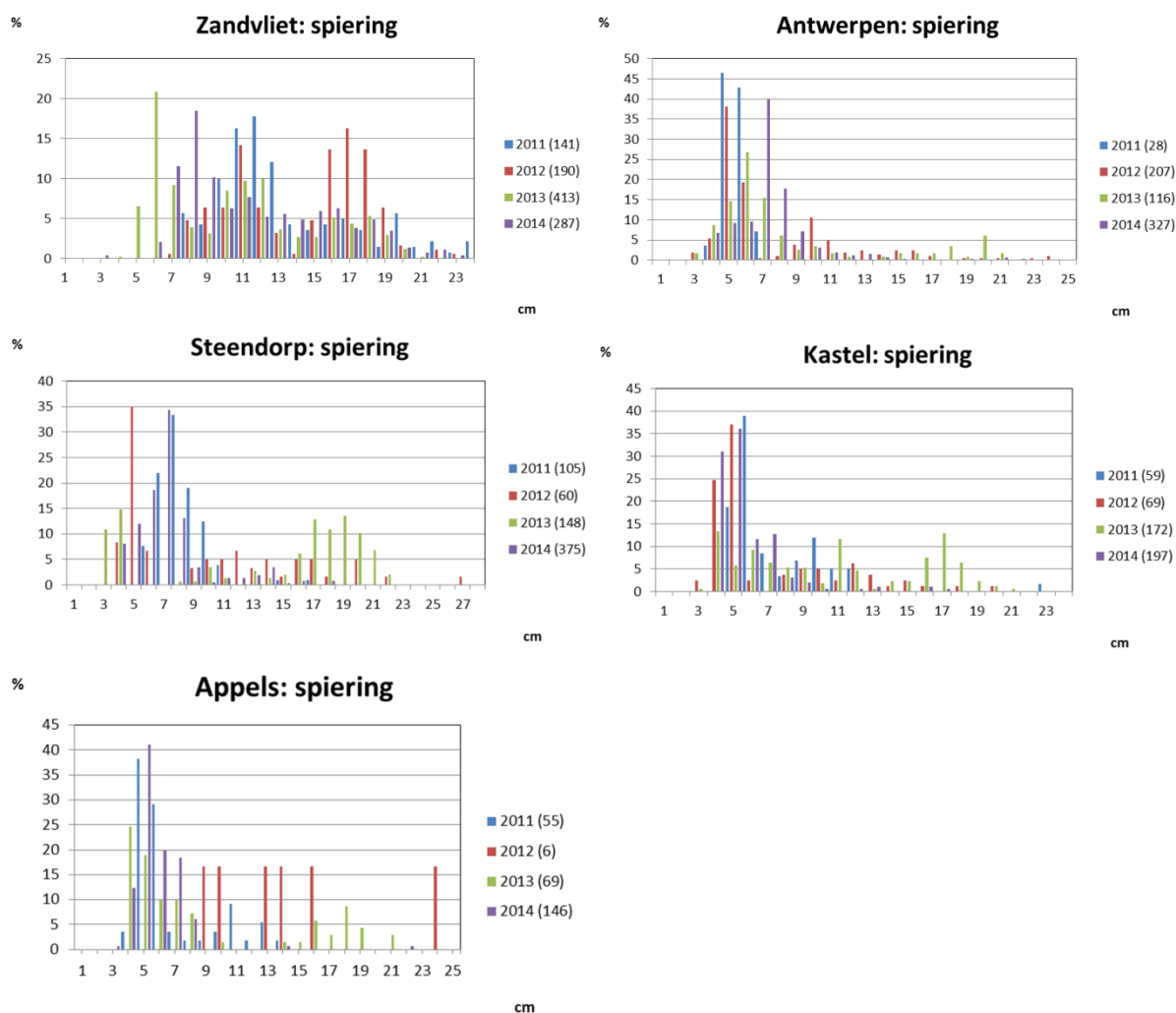
Figuur 34. Lengte frequentie (%) van spiering in vijf locaties langs de Zeeschelde (2011-2014). Het aantal gemeten exemplaren staat tussen haakjes.
