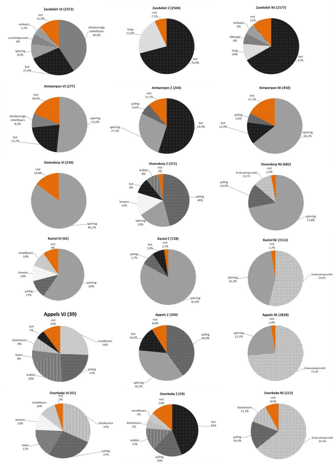
Figuur 11. Het relatief aantal gevangen individuen in de Zeeschelde tijdens de 2014 campagnes (VJ: voorjaar; Z: zomer; NJ: najaar) ( )= aantal vissen in steekproef).
