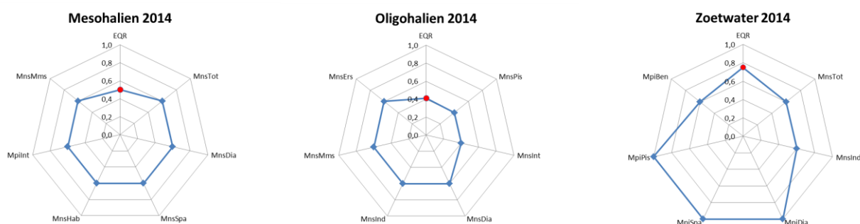
Figuur 30. Metriek scores en EQR voor de periode 2014 in de verschillende saliniteitzones van de Zeeschelde. Verklaring afkortingen zie hieronder.
