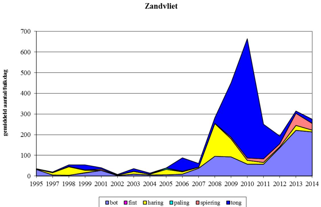
Figuur 27. Evolutie van het jaarlijks gemiddeld aantal vissen gevangen per fuik per dag voor zes indicatorsoorten ter hoogte van Zandvliet tijdens de steekproefbemonstering in het voorjaar en het najaar voor de periode 1995-2014.
