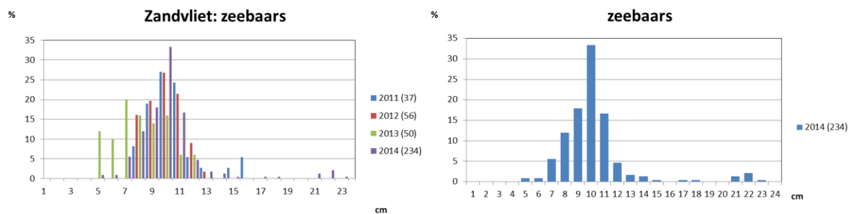
Figuur 43. Lengte frequentie (%) van zeebaars in Zandvliet (2011-2014 links en 2014 rechts). Het aantal gemeten exemplaren staat tussen haakjes.
