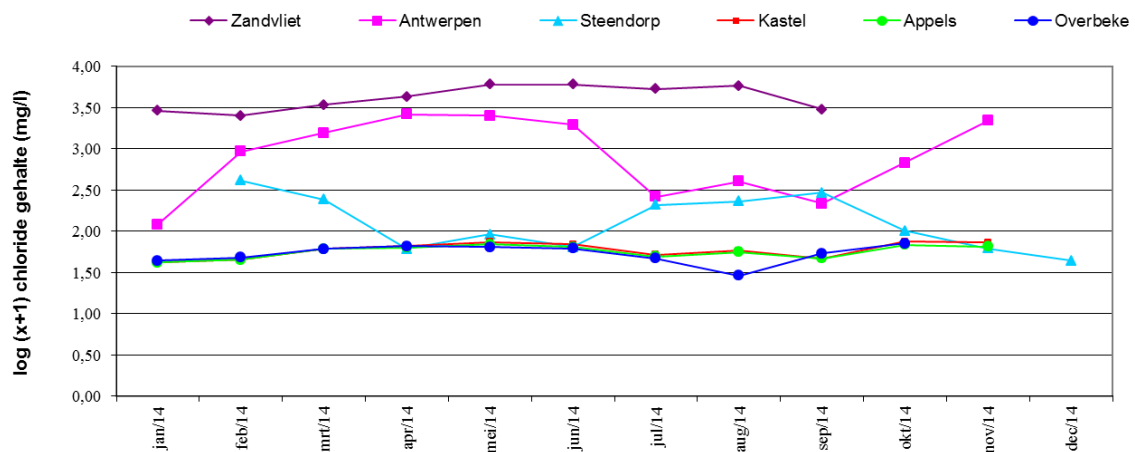
Figuur 6. Maandelijkse \log(x+1) getransformeerde waarden van het chloride gehalte ( \text{mg}/\text{l} ) op zes plaatsen in het Zeeschelde-estuarium ( www.vmm.be ; meetdatabank 2014).
