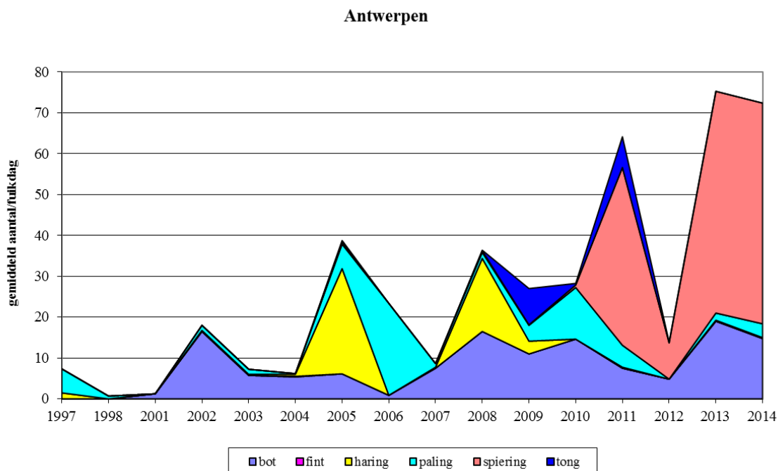
Figuur 29. Evolutie van het jaarlijks gemiddeld aantal vissen gevangen per fuik per dag voor zes indicatorsoorten ter hoogte van Antwerpen tijdens de steekproefbemonstering in het voorjaar en het najaar voor de periode 1997-2014.
