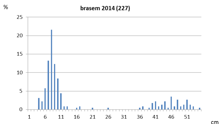
Figuur 40. Lengte frequentie (%) van brisem zes locaties van de zeeschelde (2014). Het aantal gemeten exemplaren staat tussen haakjes.
