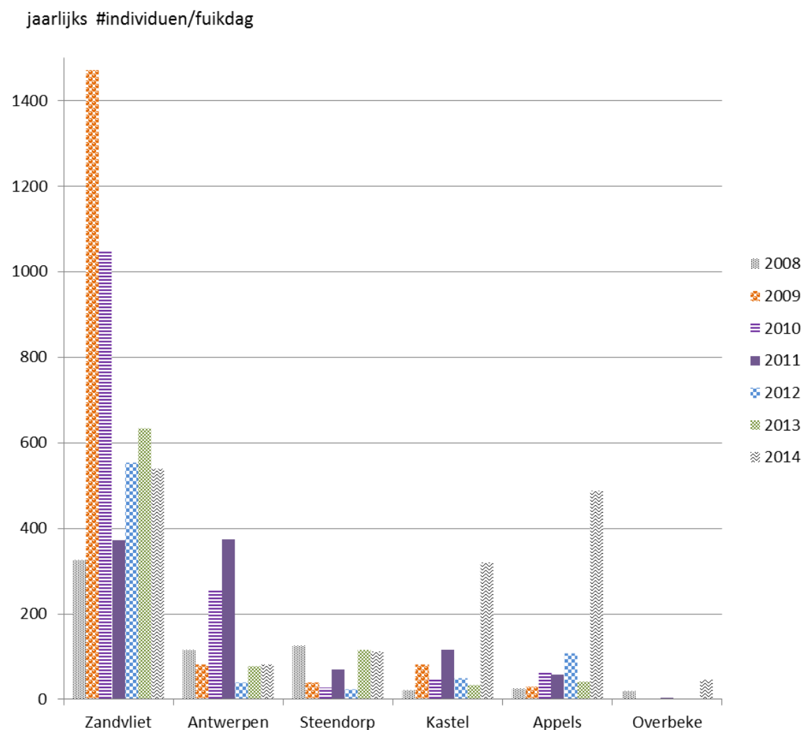
Figuur 8. Aantal individuen gevangen per fuikdag in de verschillende locaties langs de Zeeschelde (2008-2014).
