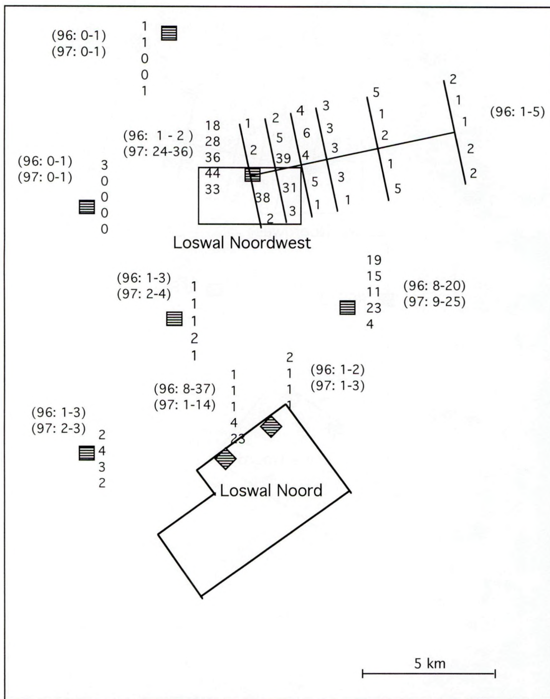
Fig. 2: Slibgehalten (fractie <63 µm, %) van het sediment op en rond Loswal Noord en Loswal Noordwest. De getallen tussen haakjes geven de range van waarden gevonden in 1996 en 1997).
