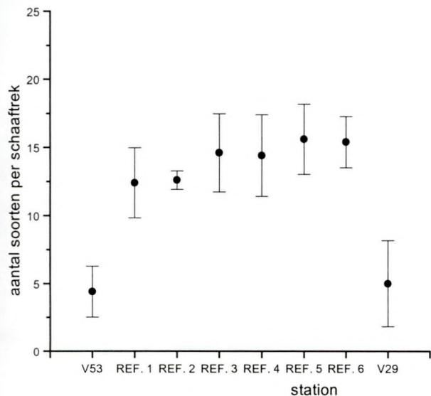
Fig. 5: Makrobenthos Loswal Noord, de referentiestations en Loswal Noordwest: Gemiddeld aantal soorten per schaaffrek en 95% betrouwbaarheidsgrenzen.
