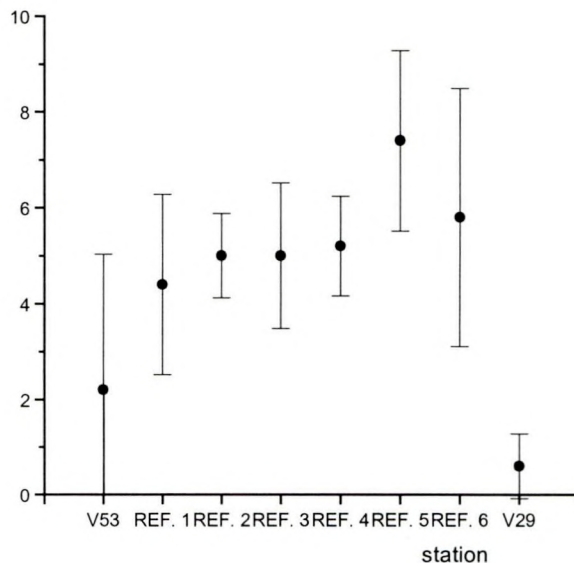
Fig. 6: Vissen op Loswal Noord, de referentiestations en Loswal Noordwest: gemiddeld aantal soorten per schaaffrek en 95% betrouwbaarheidsgrenzen.
