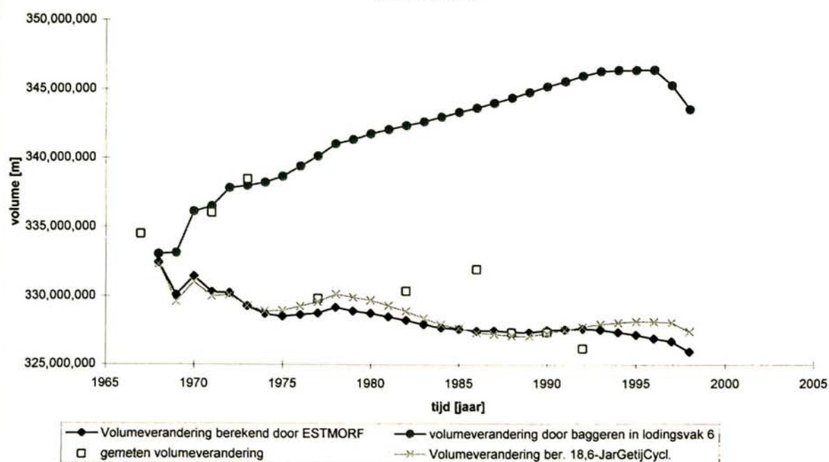
Totaaloverzicht volmume verandering lodingsvak 6 1968 t/m 1998
