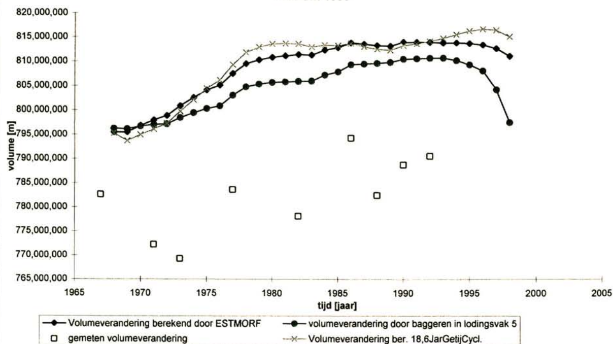
Totaaloverzicht volmume verandering lodingsvak 5 1968 t/m 1998
