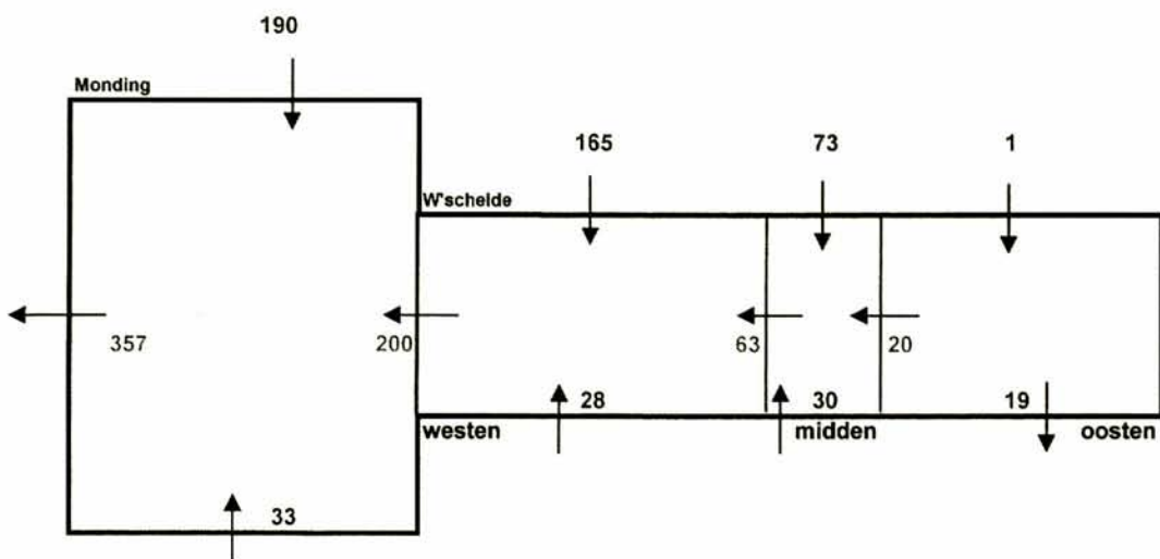
Zandbalans Mouding en de Westerschelde t.o.v. laag water
