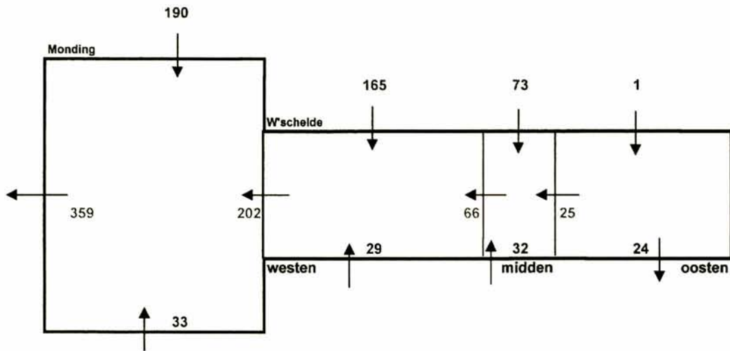
Zandbalans Mouding en de Westerschelde t.o.v. hoog water
