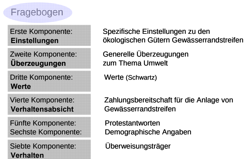
Abb. 2: Fragebogaufbau
