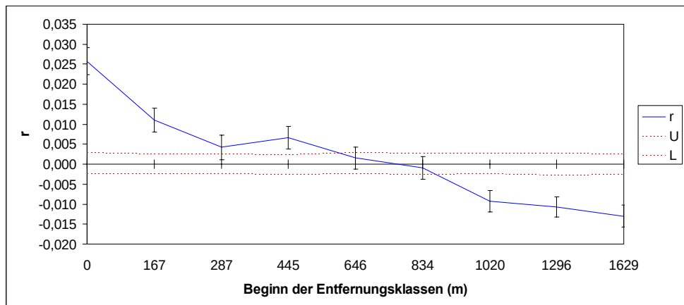
Abb. 1: Korrelogramm der räumlich- genetischen Analyse des Schwarzpappel-Altbaumbestandes. r : Korrelationskoeffizient mit Standardabweichung (schwarze Balken); U und L : untere bzw. obere Grenze des 95 % Konfidenzintervalls.
