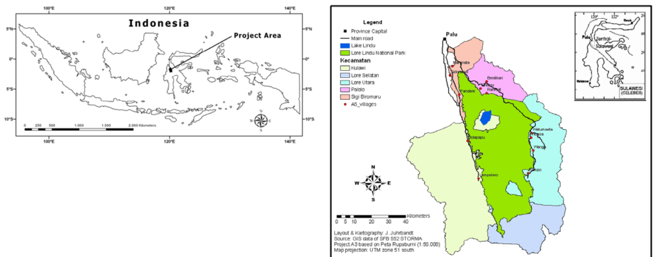
Abb. 1: Untersuchungsregion in Zentral-Sulawesi, Indonesien
