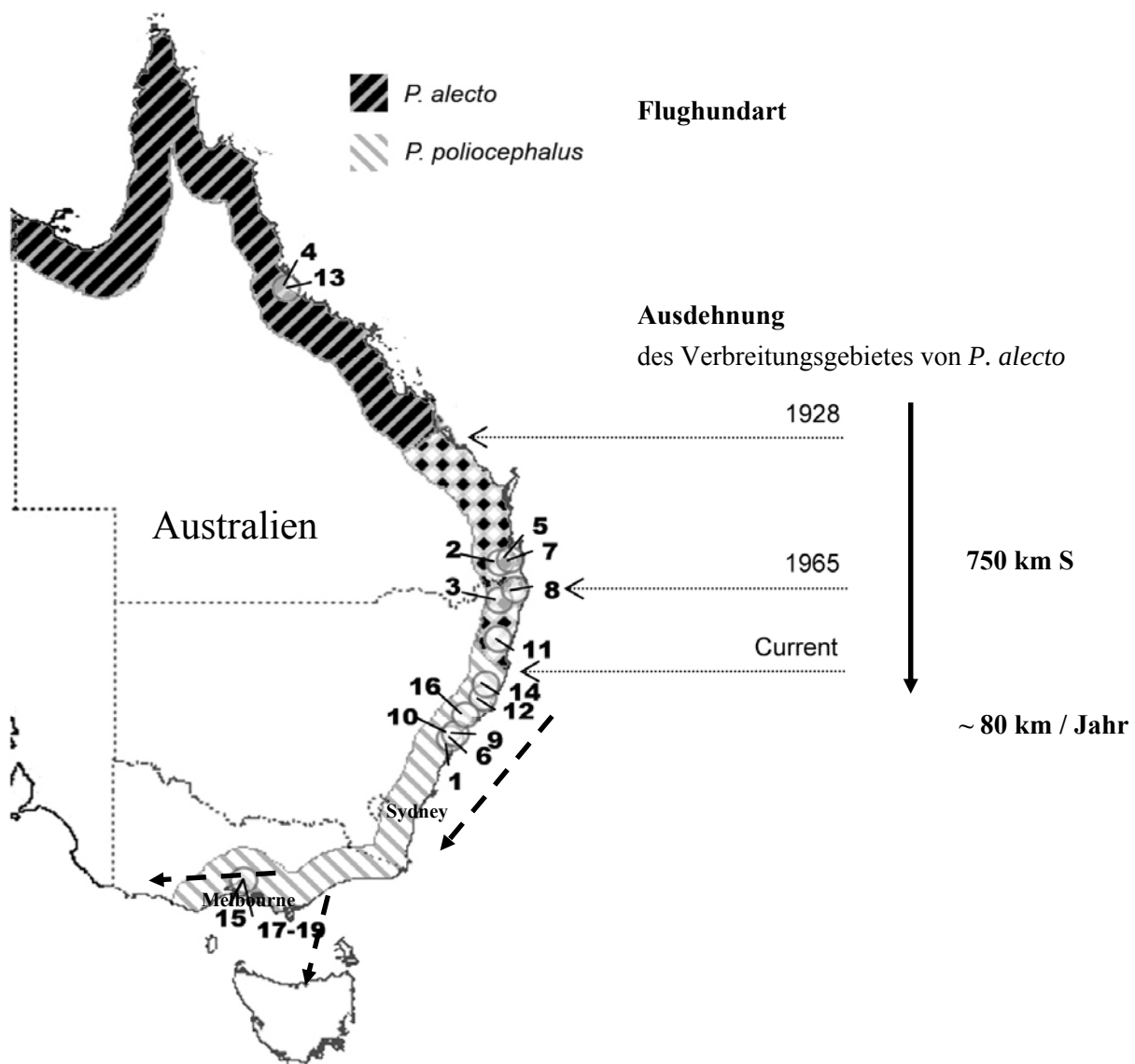
Abb. 1: Verbreitungsgebiet der beiden Studienarten entlang der australischen Ostküste. Durch die seit 1928 erfolgte Arealausweitung des Schwarzen Flughundes überlappt dessen Verbreitungsgebiet nun großflächig mit dem des Graukopfflughundes. Nummeriert sind Flughundkolonien, wo seit 1994 Massensterblichkeiten von Pteropus spp. dokumentiert worden sind (eigene Abbildung/Daten, WELBERGEN, KLOSE et al. 2008).
