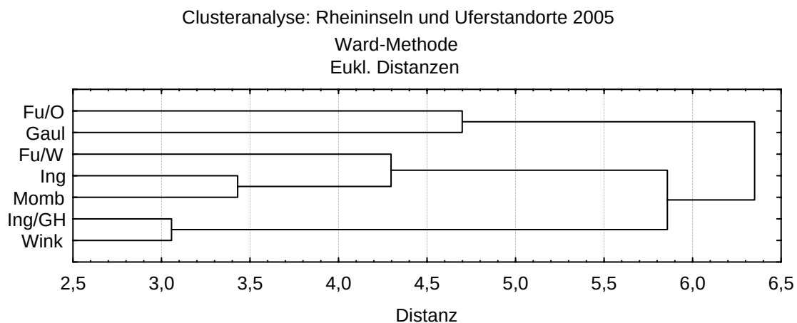
Abb. 2: Clusteranalyse der Spinnenfauna (2005) der Standorte Fulderau Ost (Fu/ O), Fulderau West (Fu/ W), Winkeler Aue (Wink), Gaulsheim (Gaul), Ingelheim hinter dem Damm (Ing/ GH), Ingelheim vor dem Damm (Ing) und Mainz-Mombach (Momb). Eine Trennung zwischen den Faunen der Rheininseln und der Uferstandorte ist nicht möglich.
