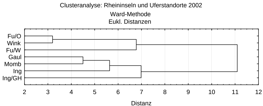
Abb. 1: Clusteranalyse der Spinnenfauna (2002) der Standorte Fulderau Ost (Fu/ O), Fulderau West (Fu/ W), Winkeler Aue (Wink), Gaulsheim (Gaul), Ingelheim hinter dem Damm (Ing/ GH), Ingelheim vor dem Damm (Ing) und Mainz-Mombach (Momb). Anhand der Faunenähnlichkeit bilden die Rheininseln und die Uferstandorte eigene Cluster.
