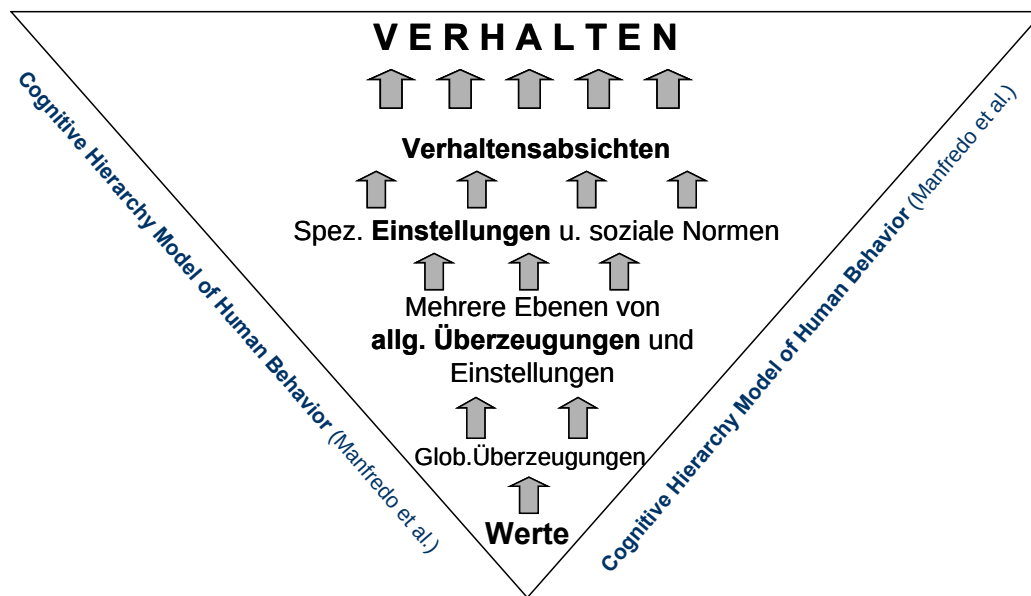
Abb. 1: Verhaltensmodell
