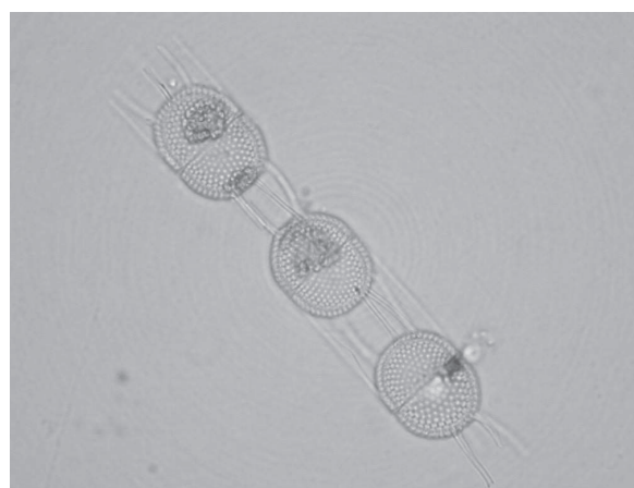
Figura 2. Células de Stephanopyxis nipponica . Diámetro: 25 µm; areolas: 6 en 10 µm; espinas: 4-5 por valva.
