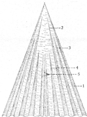
Fig. 3. — Cyrtospirifer bisinus (H. LE HON). Formule sinale.
