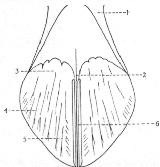
Fig. 4. — Cyrtospirifer bisinus (H. LE HON).
