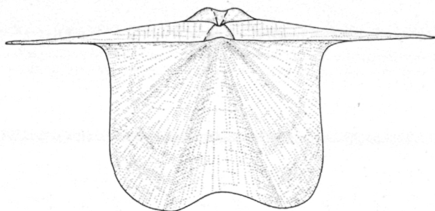
Fig. 2. — Reconstitution du Holotype de Cyrtospirifer malaisei avec ses mucronations cardinales.
