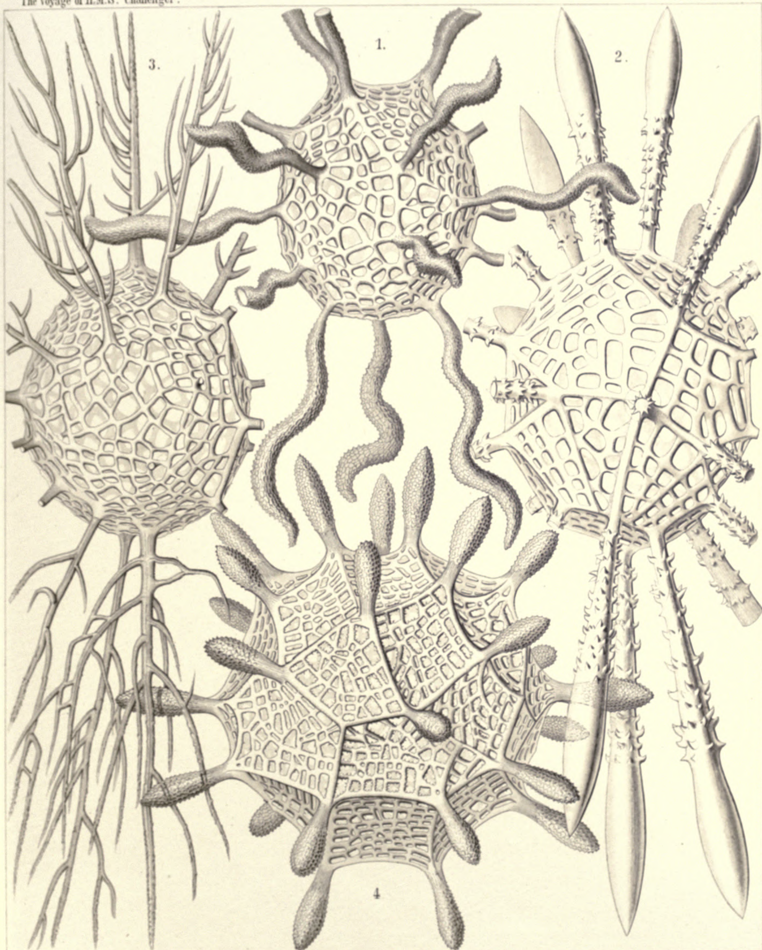
1. 2. ORONIA, 3. OROTHAMNUS, 4. OROSCENA.
