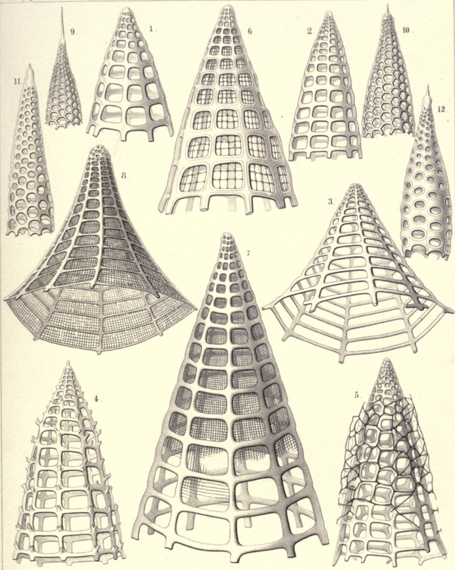
1-4. BATHROPYRAMIS, 5. PERIPYRAMIS, 6-8. CINCLOPYRAMIS, 9-12. CORNUTELLA.
