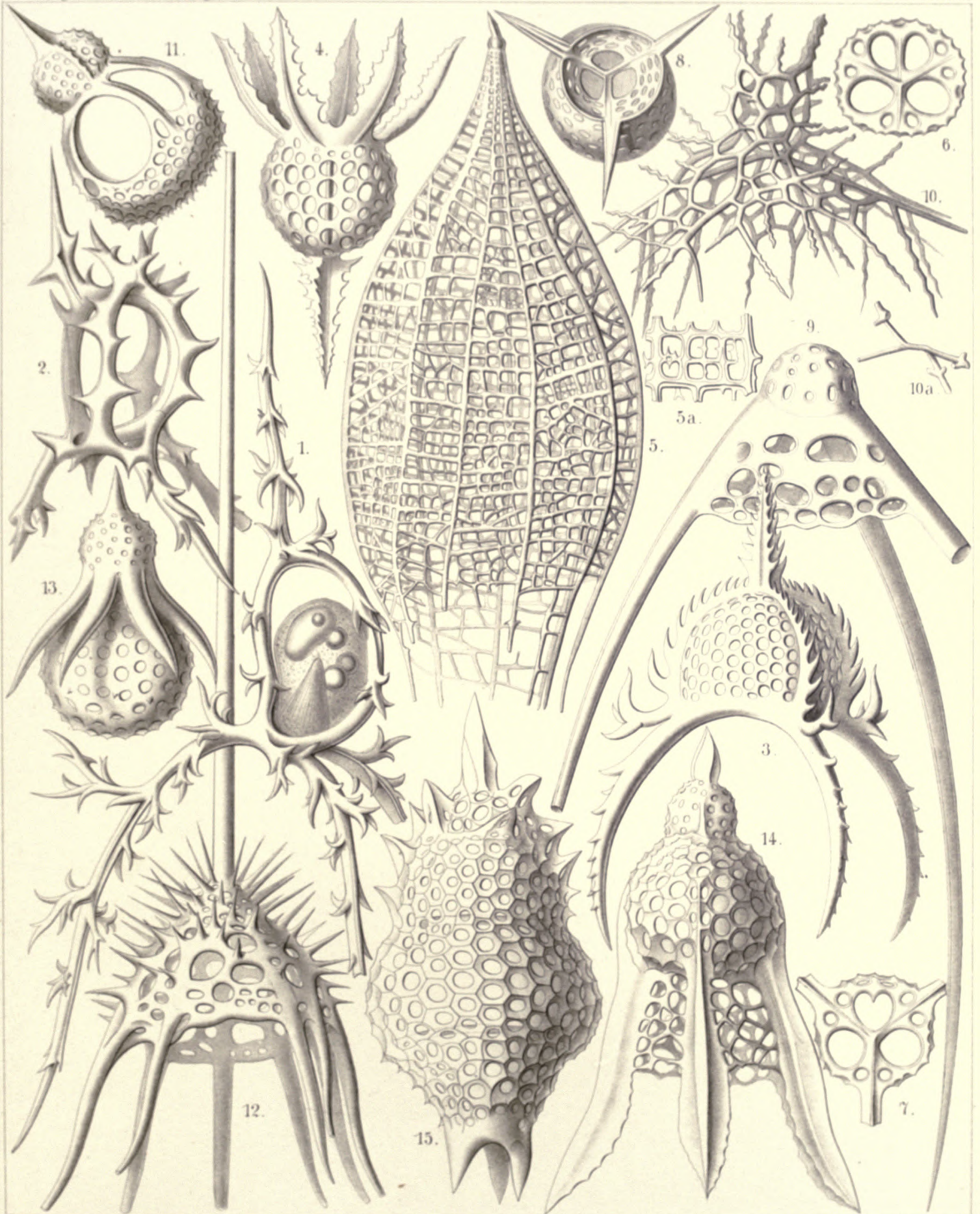
1, 2. CORTINA. 3-7. MONOCYRTIDA. 8-13. DICYRTIDA. 14. THEOPODIUM. 15. PODOCAMPE.
