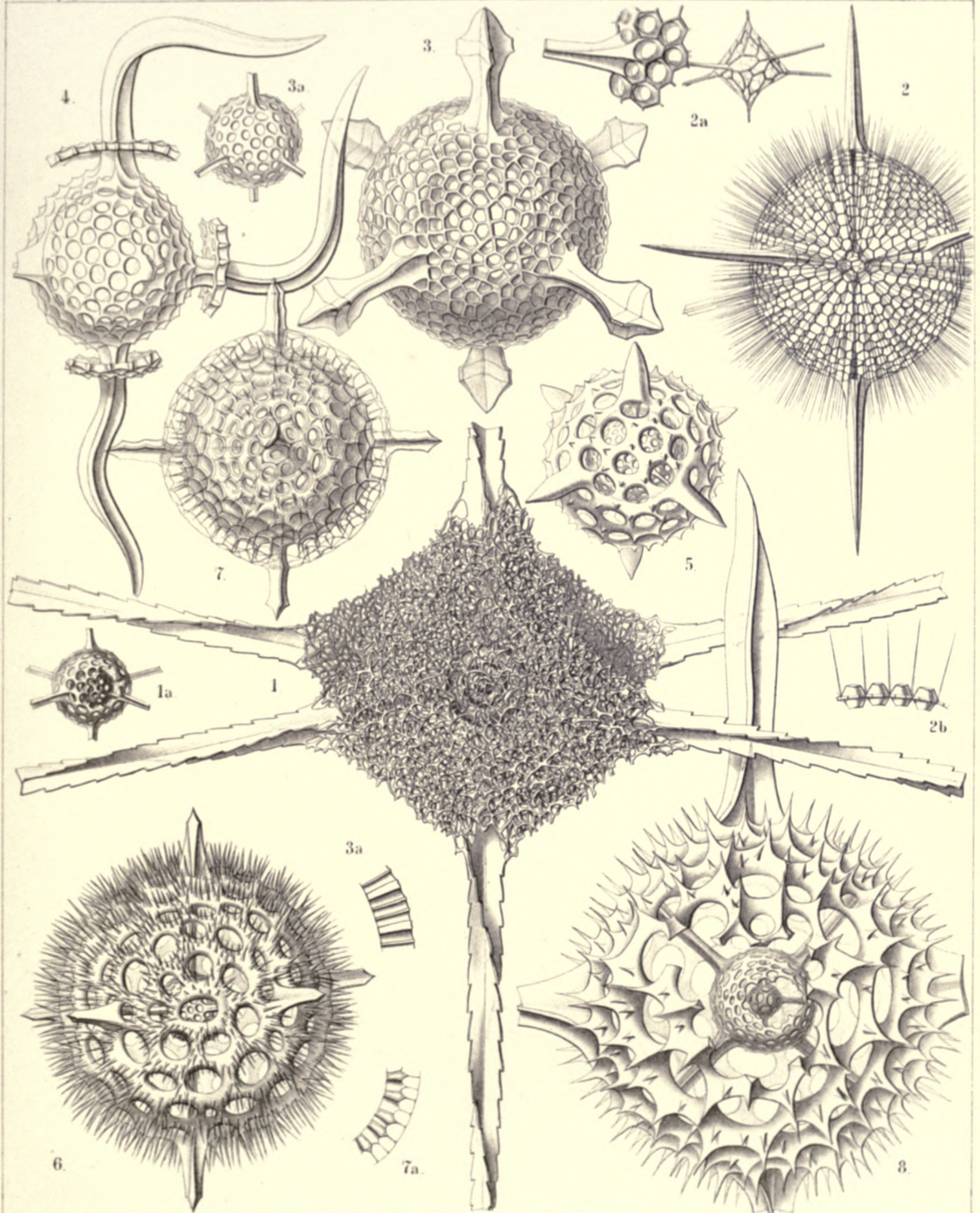
1. HEXADORAS, 2-6. HEXALONCHE, 7 & 8. HEXACONTIUM.
