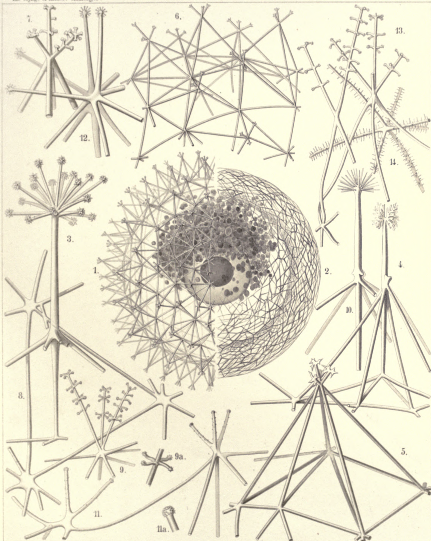
1-7. SAGOSCENA, 8. SAGENA, 9-14. SAGOSPHERA.
