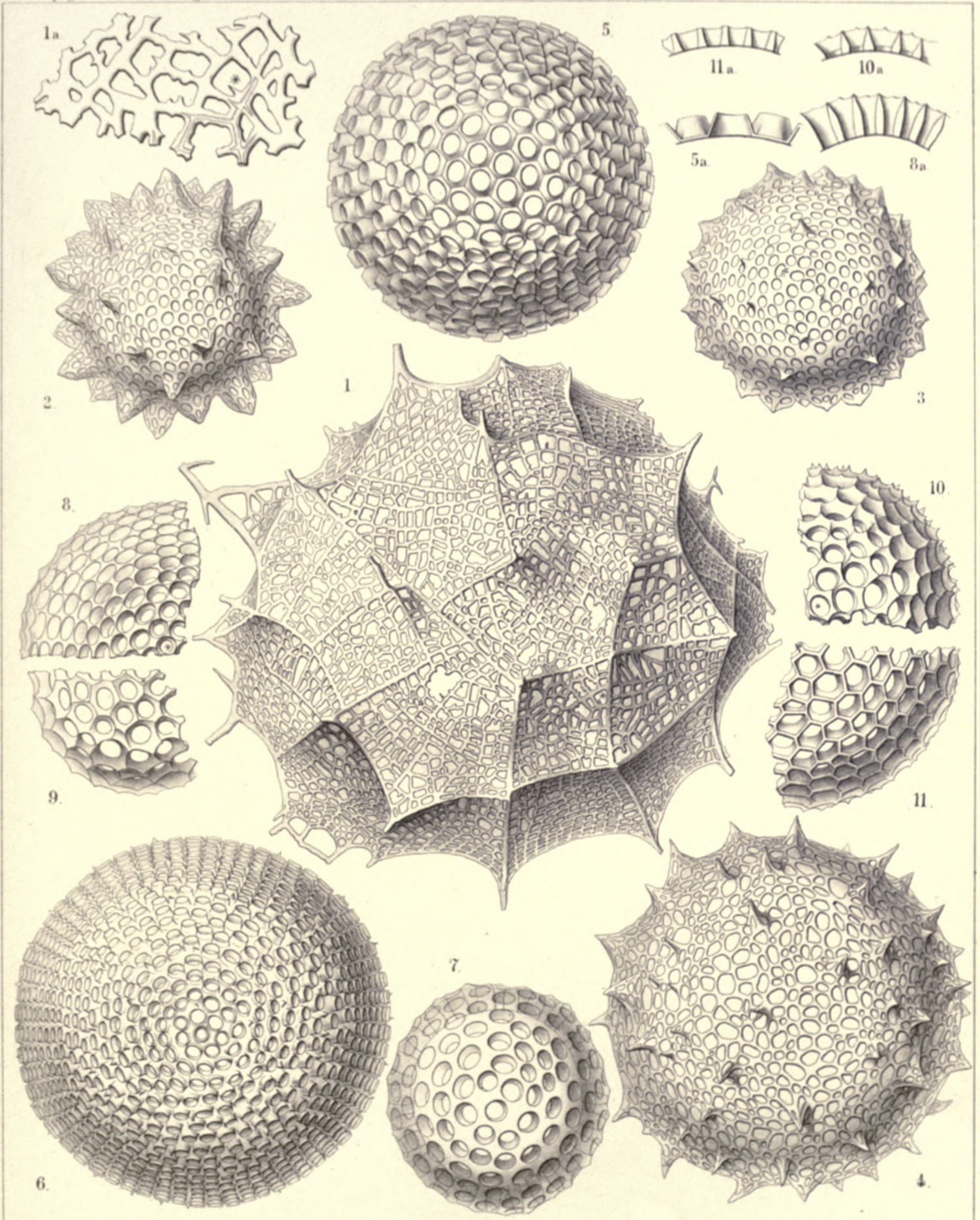
1. OROSPHAERA, 2-4. CONOSPHERA, 5, 6. ETHMOSPHERA, 7-11. CERIOSPHERA.
