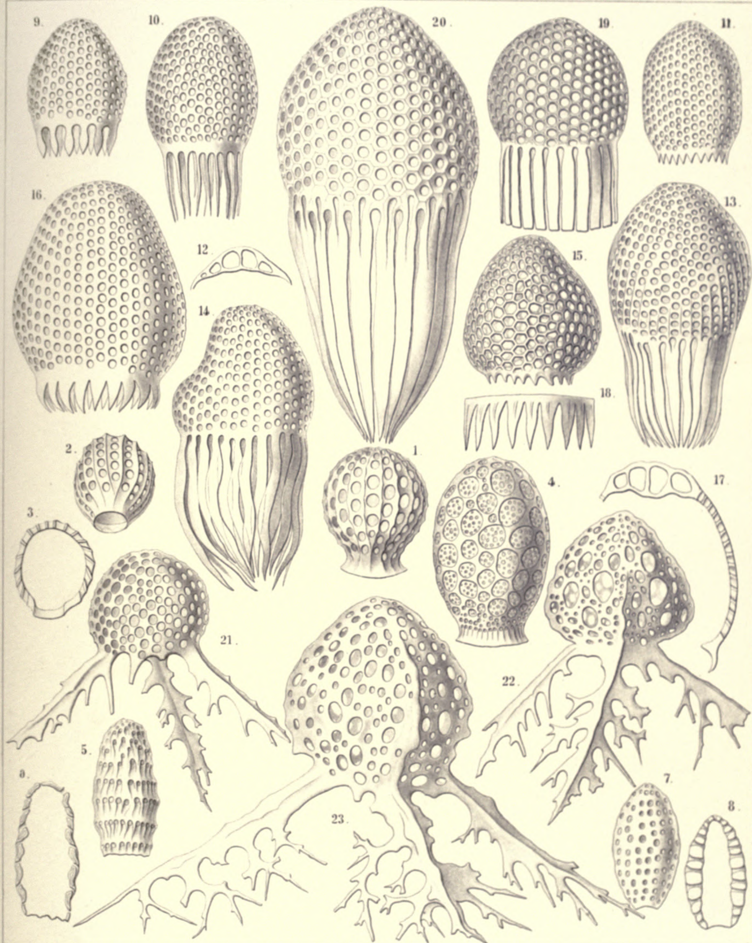
1-8. CYRTOCALPIS. 9-20. CARPOCANIUM. 21-23. TRIPODISCIMUM.
