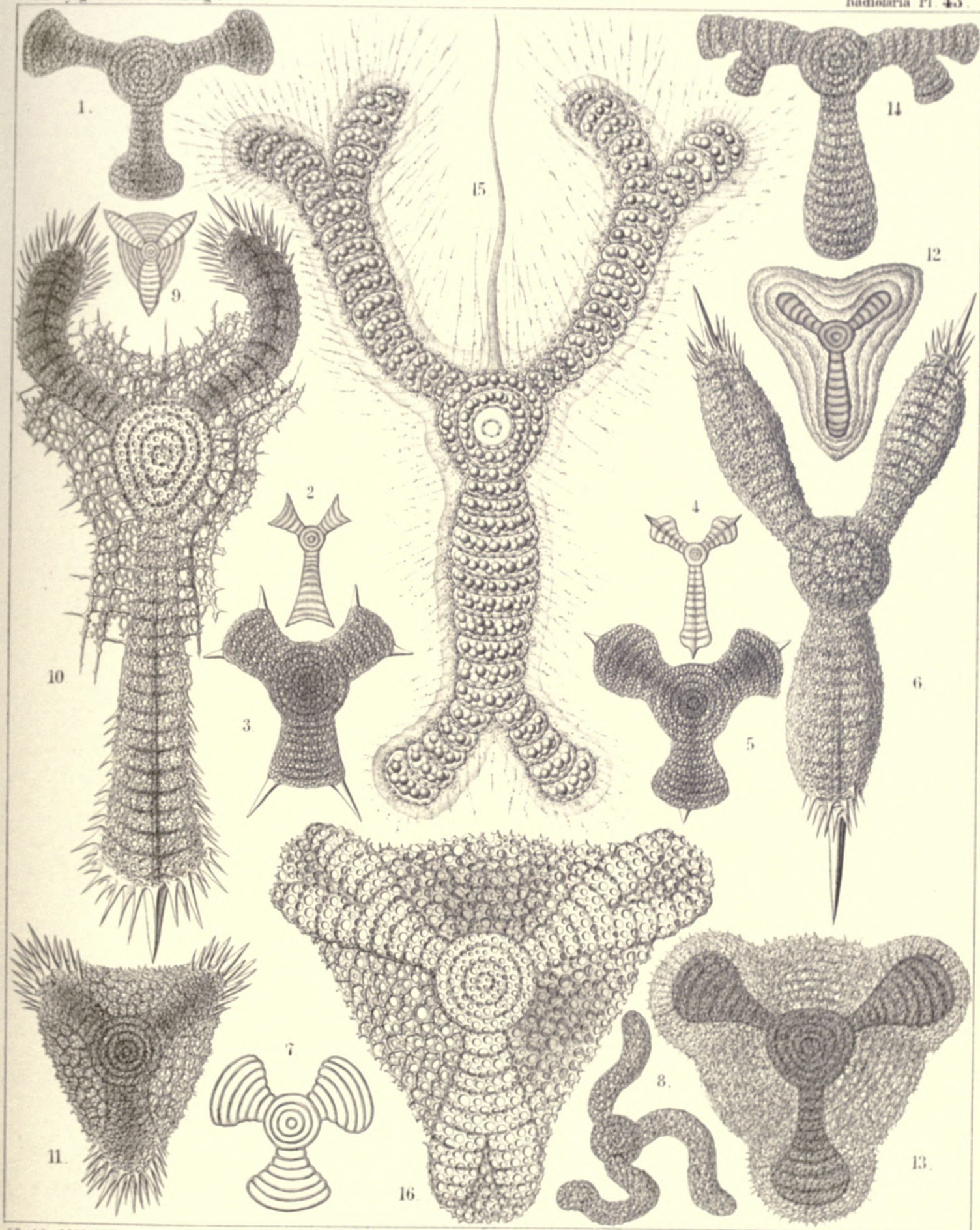
1-8. RHOPALASTRUM, 9-11 HYMENIASASTRUM, 12 13 EUCHITONIAS. 14 15 DICTYASTRUM, 16 CHITONIASASTRUM.
