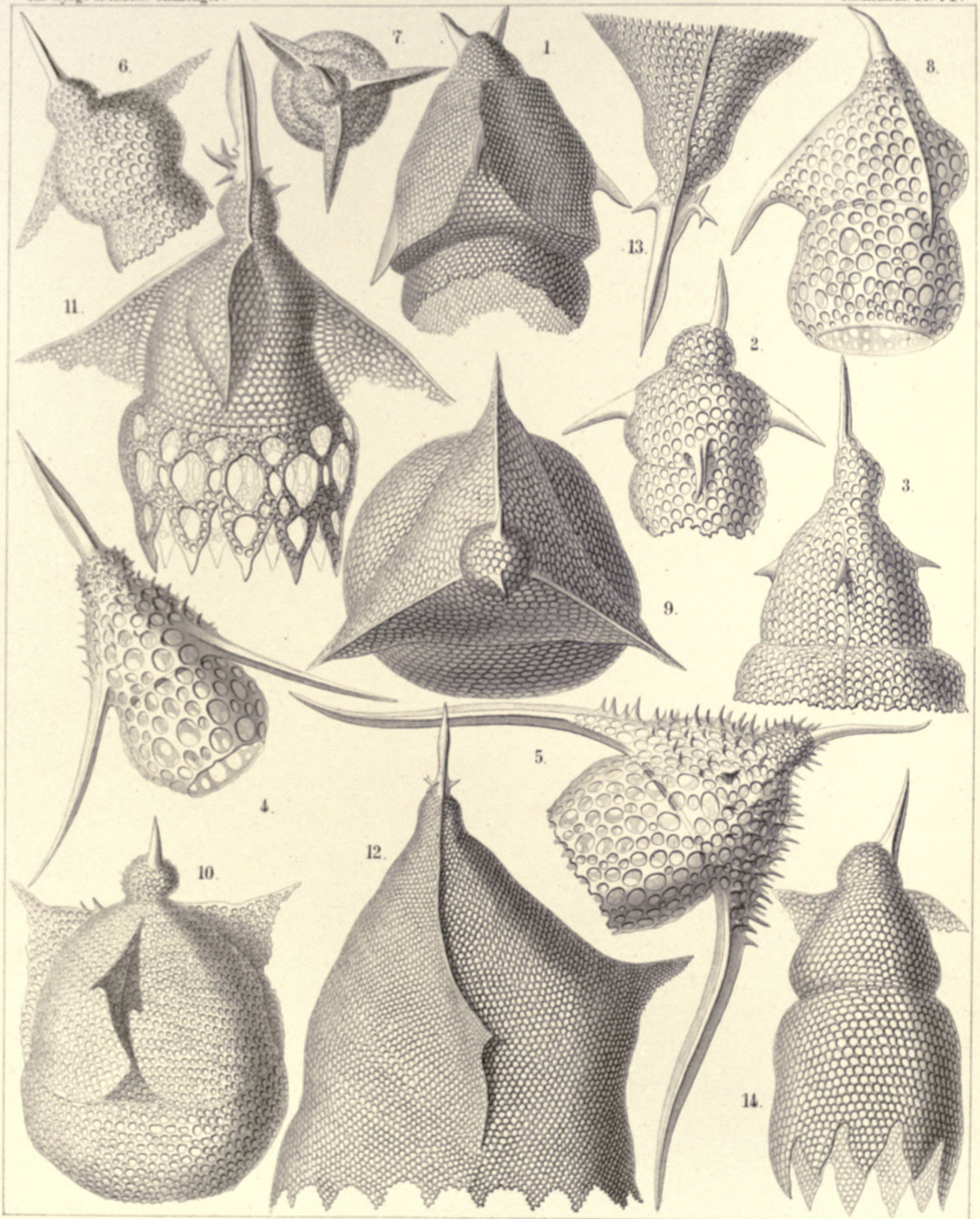
1-5. PTEROCORYS, 6-10. DICTYOCERAS, 11-14. DICTYOCODON.
