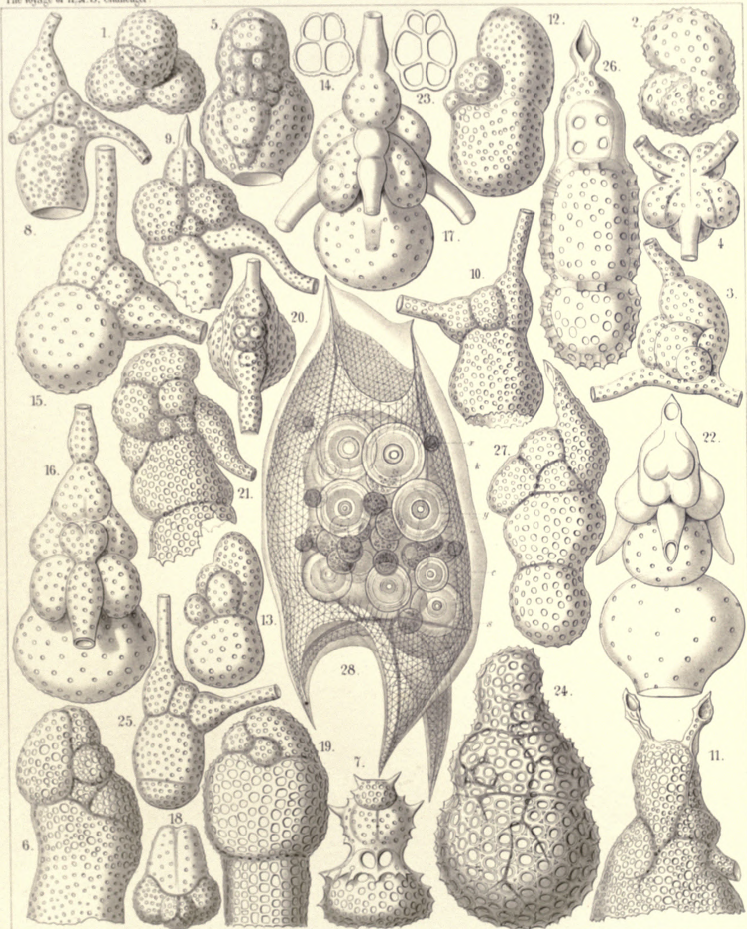
1-4 BOTRYOPERA, 5-11. BOTRYOPYLE, 12-17. BOTRYOCELLA, 18-22. BOTRYOCYRTIS, 23-27. BOTRYOCAMPE, 28. CEPHALOSPYRIS.
