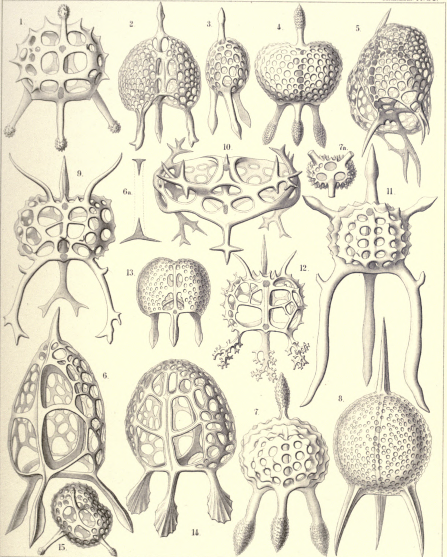
1-8. TRIPODOSPYRIS , 9-12. TRICERASPYRIS , 13-15. TRISTYLUSPYRIS
