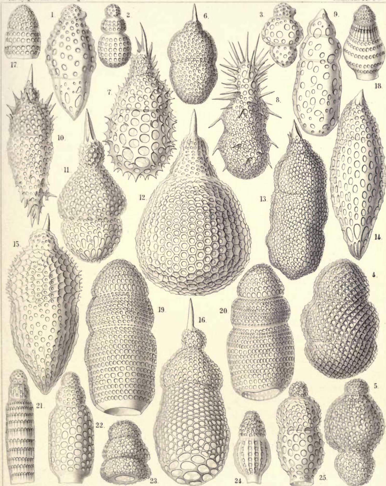
1-5 TRICOLCAPSA, 6-16, TRICOLPERA, 17-25 TRICOLCAMPE.
