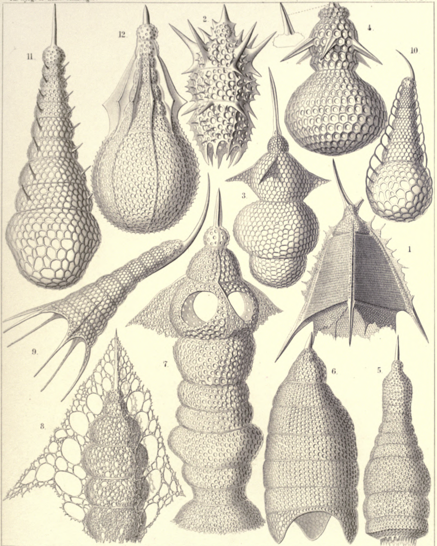
1 ARTOPILIUM, 2 ARTOPHORMIS, 3 ARTOPERA, 4 ARTOPHATNA, 5 STICHOCORYS, 6 STICHOPODIUM, 7 CLATHROPYRGUS, 8 STICHOPTERYGIUM, 9 STICHOFORMIS, 10 CYRTOLAGENA, 11 STICHOPERA, 12 STICHOPHATNA.
