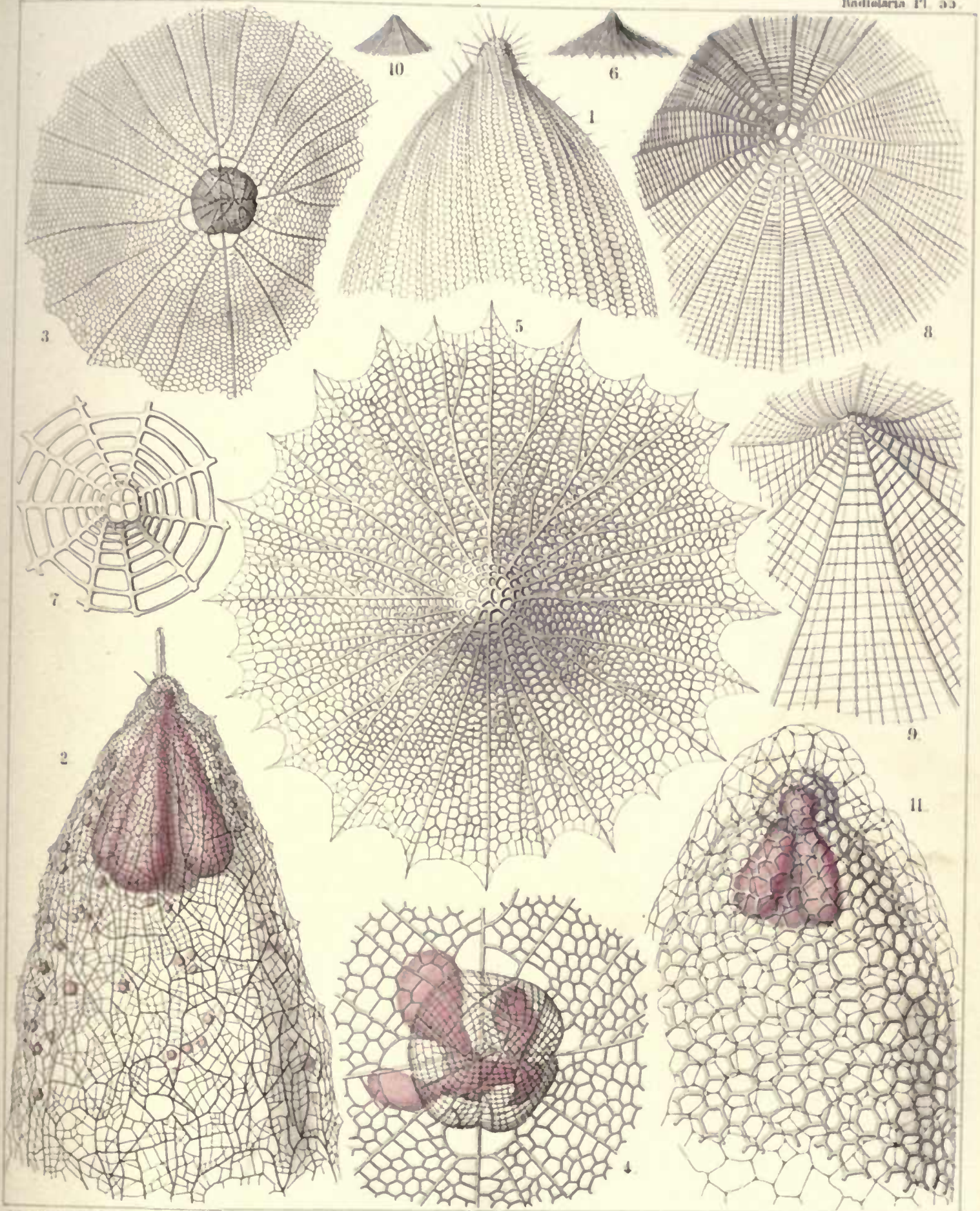
1 2 PHLEBARACHNIUM. 3 4 LEPTARACHNIUM. 5 10 LITHARACHNIUM. 11 PERIARACHNIUM.
