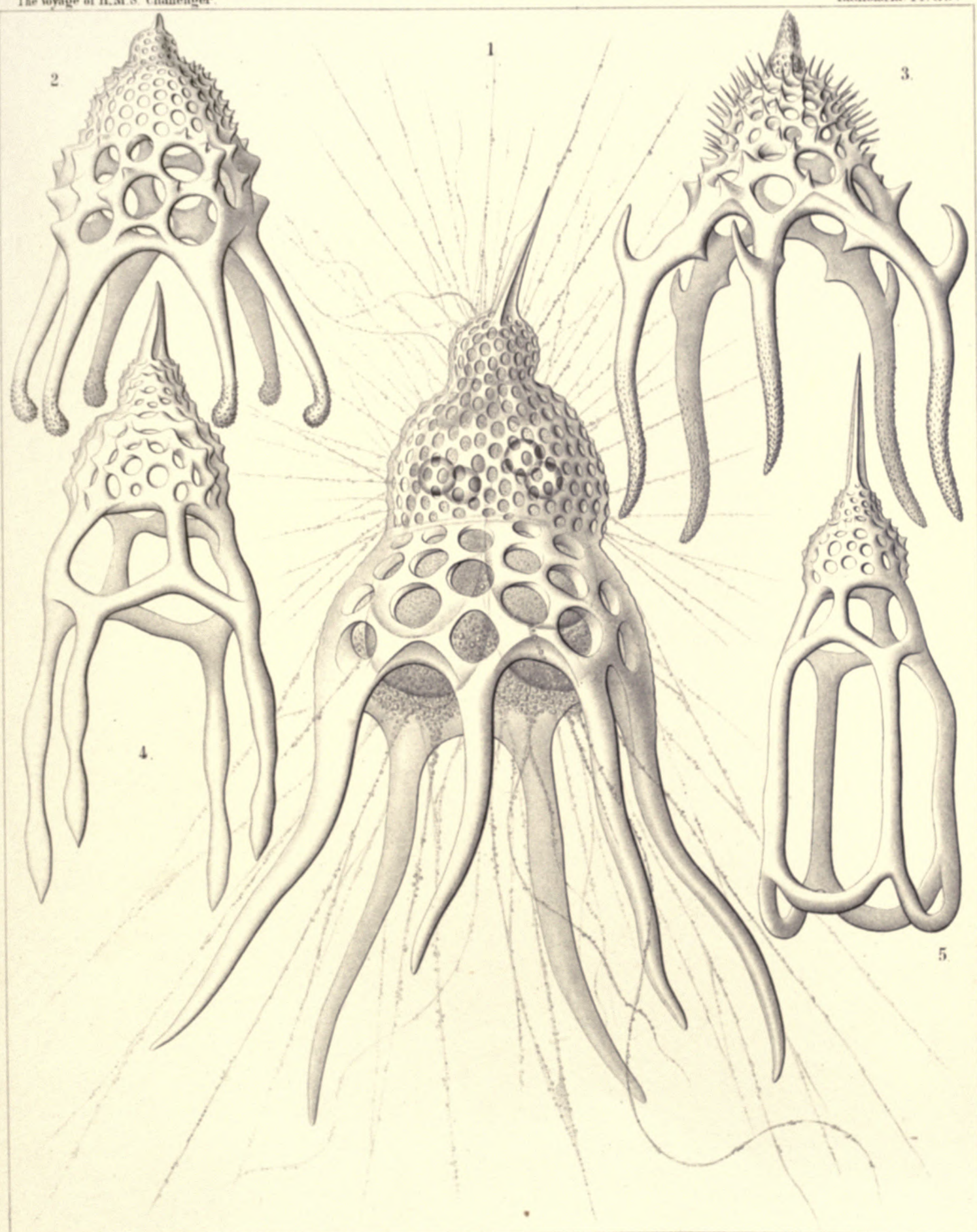
1 2 HEXALACORYS, 3 PENTALACORYS, 4 TETRALACORYS, 5. THEOPHORMIS.
