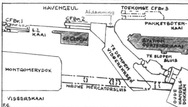
Fig. nr. 219. Haven Oostende, 1971. Overzichtstekening van de werken voor de bouw van de Mercator-sluys en het vormen van uitbreiding carferryterminal en stationsplein.
