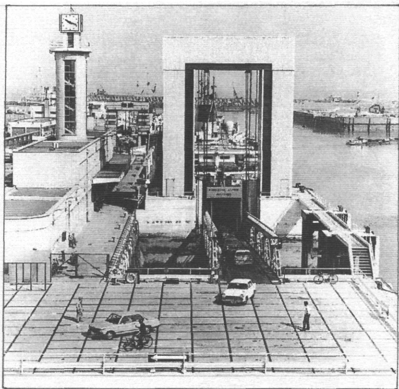
Fig. nr. 215. Haven Oostende, 1971. Carferrybrug 2, ontscheping van voertuigen uit het m.s. Princesse Astrid. Op de voorgrond het landhoofd, gedeeltelijk gebouwd in de monding van de Visserskreek. Links het Carferrygebouw.
