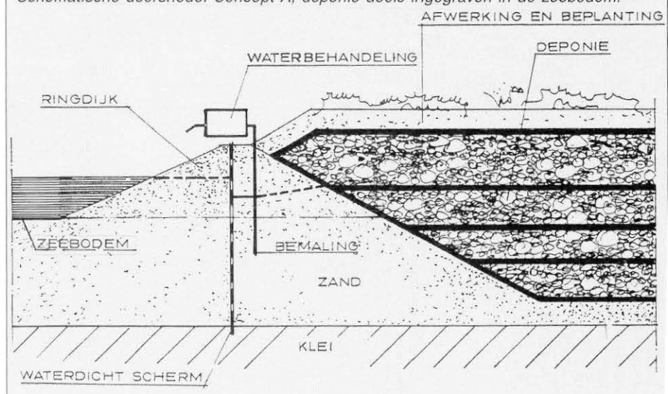
Schematische doorsnede. Concept A, deponie deels ingegraven in de zeebodem.
