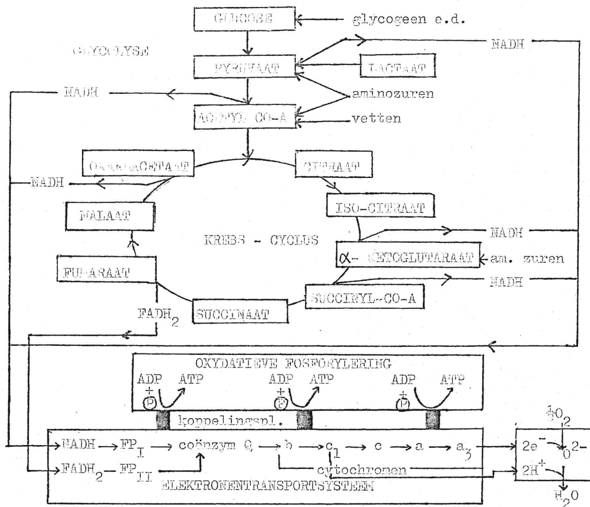
Fig. 1 : De elektronentransportketen der oxydatieve fosforylering en zijn relatie tot de Krebs-cyclus en de glycolyse. (gewijzigd naar PACKARD 1971), (FP = flavoproteïne systeem)
