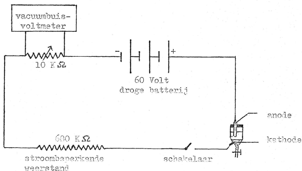
Fig. 2 : Schakelschema gebruikt bij het iken van de IMT-onlossingen. (gewijzigd naar PACKARD & FRARY 1958).
