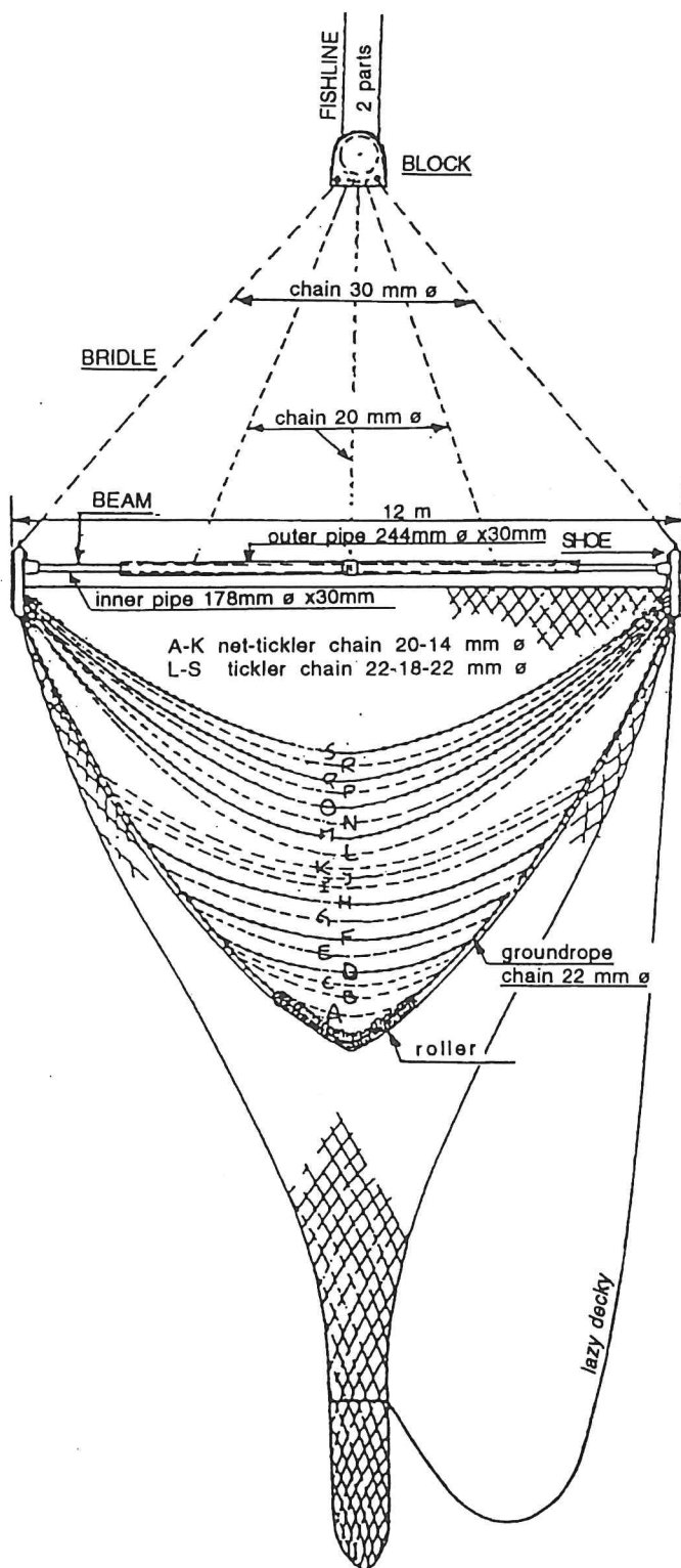
Fig. 3a. Beamtrawl-gear
