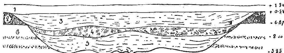
Fig. 1. — COUPE AB DE LA PLANCHE XX.
