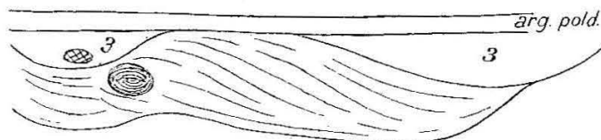
Fig. 5. — COUPE AU POINT D. Schéma de la photo fig. 6.
