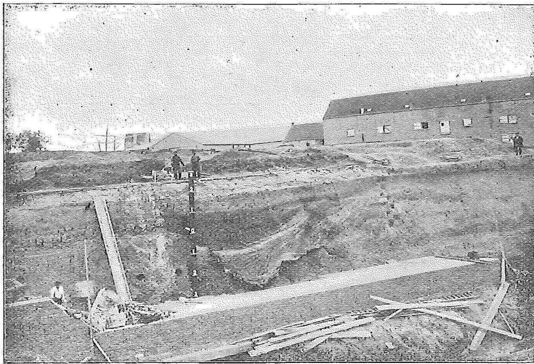
Fig. 8. — PHOTOGRAPHIE DE LA TRANCHEE REPRÉSENTÉE SUR LE SCHÉMA B DE LA FIGURE 7. (Fig. 2, BASSIN D.)
