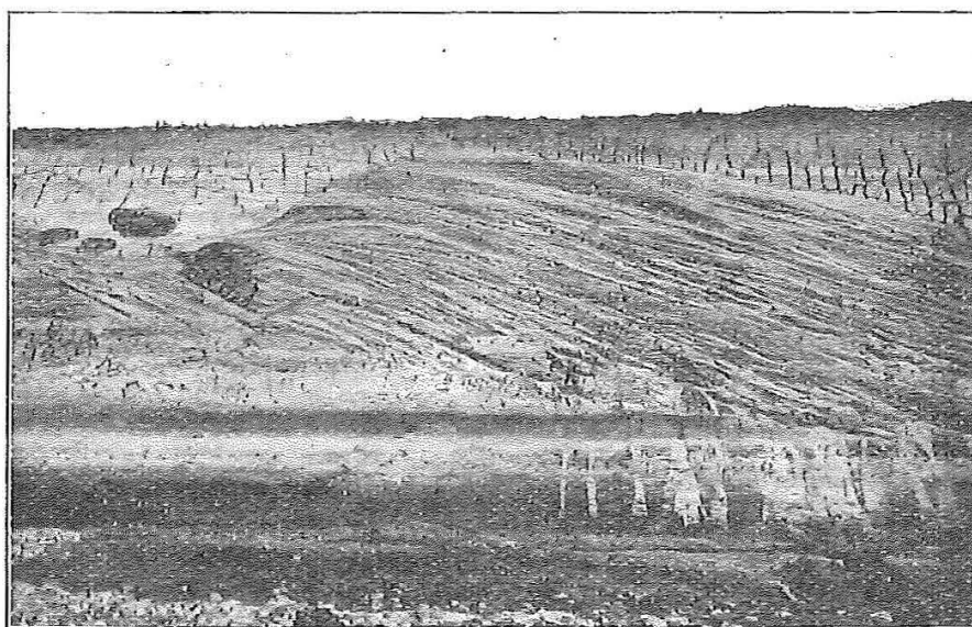
Fig. 6. — PHOTO AU POINT D.
