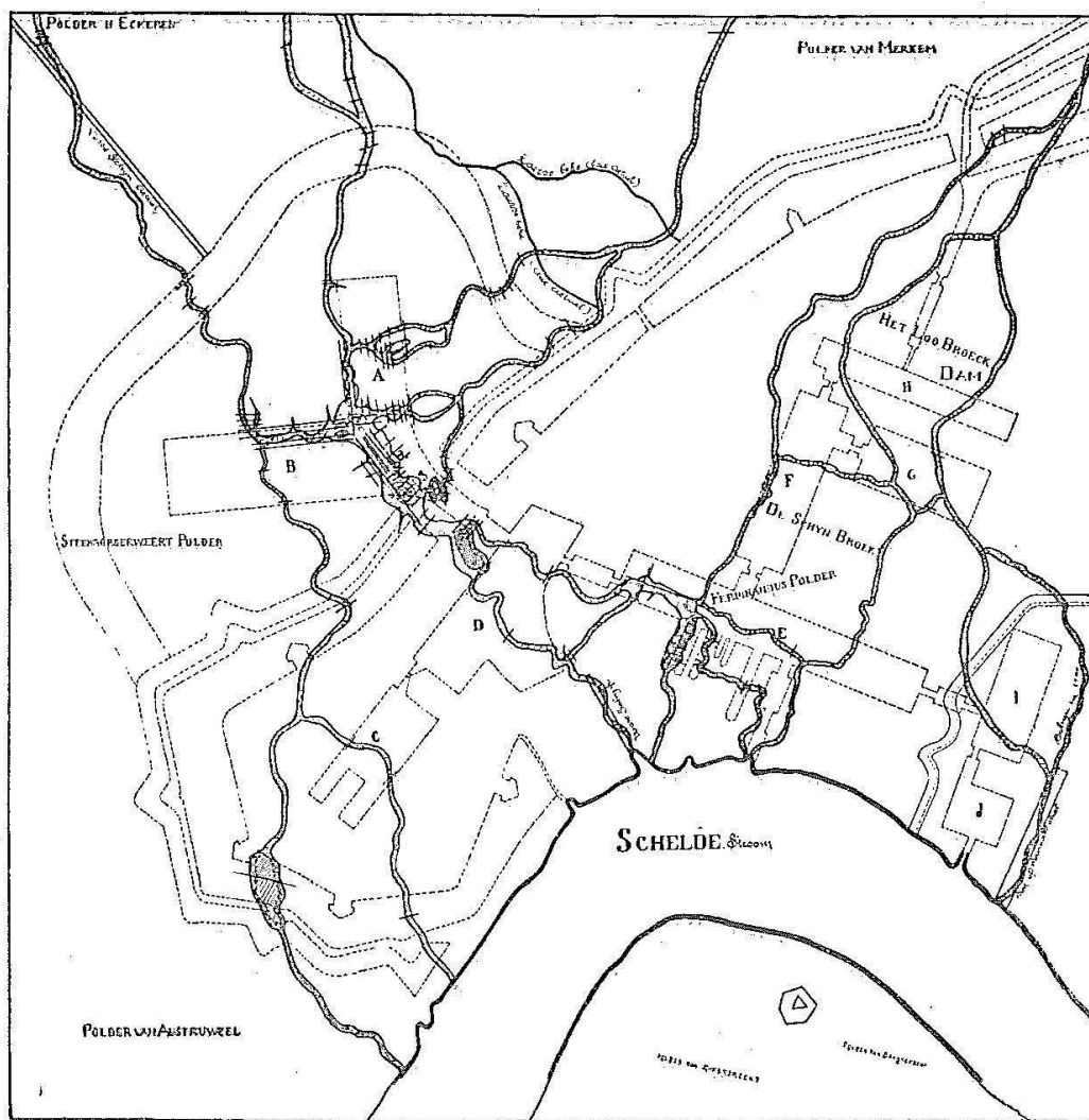
Fig. 2. — RECONSTITUTION DU COURS DES SCHIJNS AU NORD D'ANVERS.
