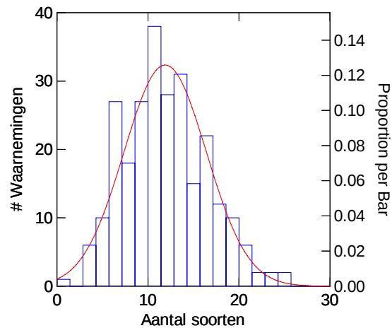
Figuur 17 Frequentieverdelingen van de waarnemingen voor het aantal soorten bodemdieren. De bijbehorende normale verdeling (met zelfde gemiddelde en spreiding als de waarnemingen) is weergegeven in de grafiek.
