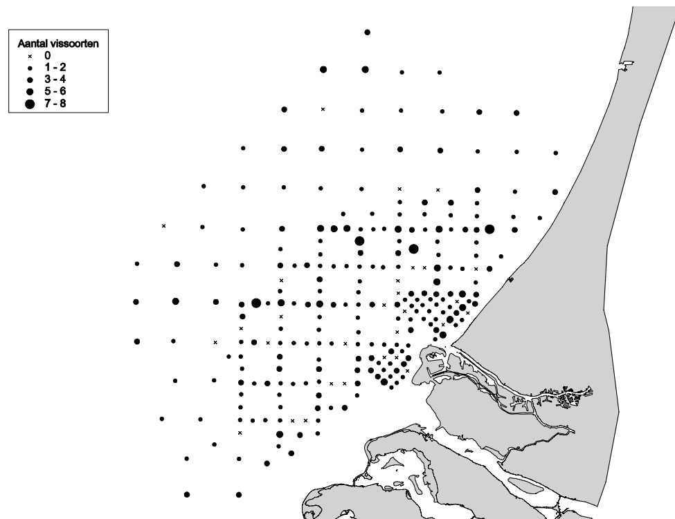
Figuur 15 Aantal soorten vis per schaaftrek.
