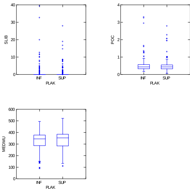
Figuur 3 “Box and whisker” plots van de waarnemingen voor het slib gehalte (SLIB, %), de concentratie in organische stof (POC, %), en de mediane korrelgrootte (MEDMU, \mu\text{m} ) als functie van de bemonsteringstrata INF (0-5cm) en SUP (5-10 cm).
