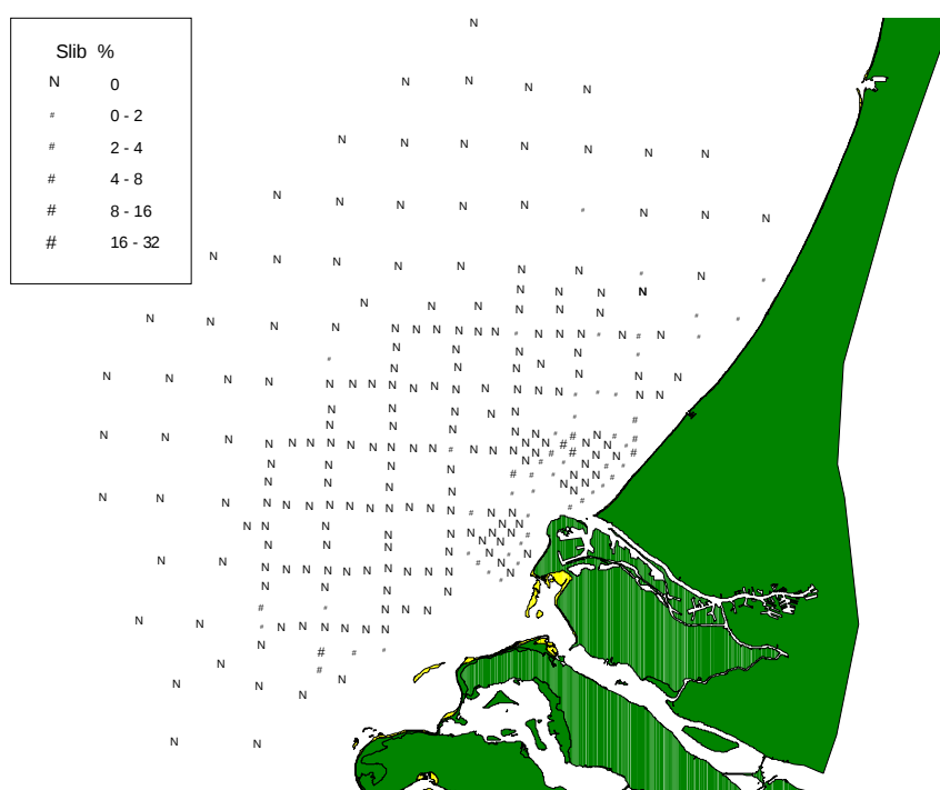
Figuur 9 Slib gehalte (%) van de sedimentmonsters in het onderzoeksgebied.
