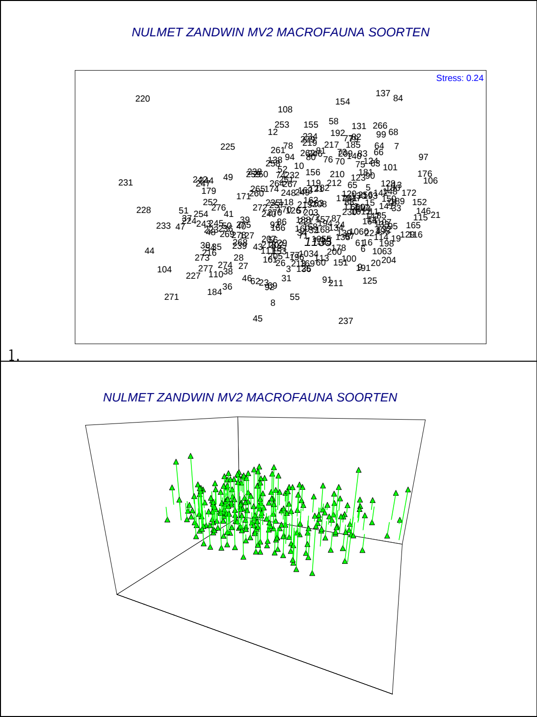
Bijlage 5 2D en 3D MDS plot van de gelijkenis matrix (Bray Curtis coefficient) berekend tussen de monsterpunten op basis van de dichtheden (vierde wortel getransformeerd) van de 34 soorten aanwezig in meer dan 10% van alle monsters (Bijlage 4).
