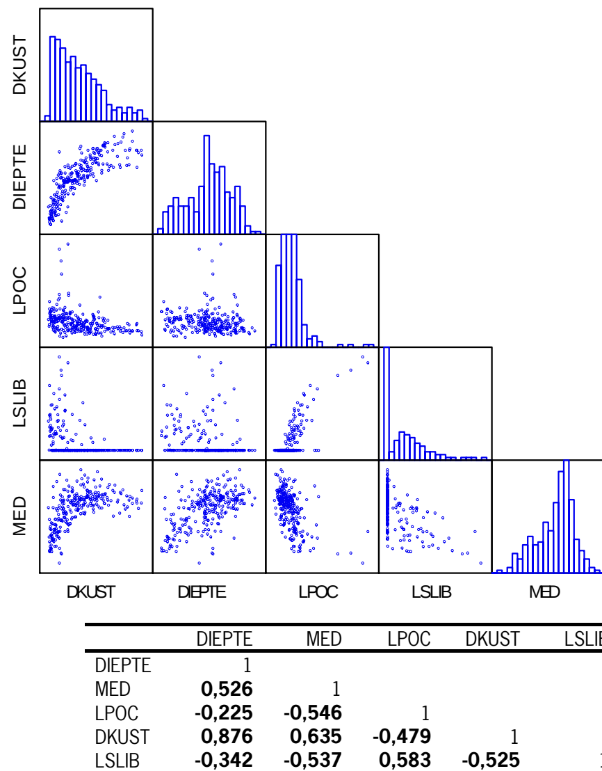
Figuur 6 Boven: Verdeling van de omgevingsvariabelen sediment (MED, POC en SLIB), diepte en afstand tot de kust (DKUST) en hun onderlinge relatie. De waarden van slib en organisch gehalten zijn log-getransformeerd (LSLIB, LPOC). Onder: Spearman rangcorrelatie matrix tussen de variabelen (significante correlaties ( p < 0,01 ) zijn vet afgedrukt).
