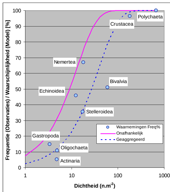
Figuur 22 Aanwezigheid van de dominante taxonomische groepen tegenover de waargenomen dichtheden (Punten). Trefkans als functie van de dichtheid voorspeld door de Poisson verdeling voor monsteroppervlak gelijk aan 0,077m 2 (ononderbroken lijn). Voorspellingen voor een individuele aggregatie (x3) van de organismen (gebroken lijn).
